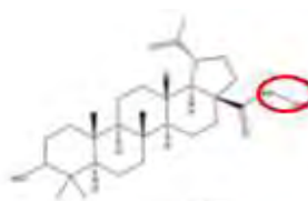
Δομή παραγώγου #15 βετουλινικού οξέος
