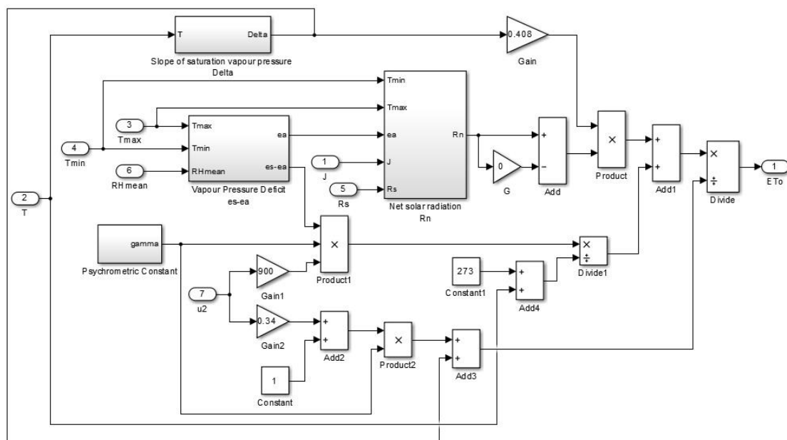
Εικόνα 5.7. Μοντέλο της εξατμισοδιαπνοής αναφοράς κατά Penman-Monteith
