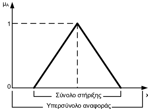
Εικόνα 3.13. Παράδειγμα τριγωνικού ασαφούς συνόλου (Κινγκ, 2004, fig. 5.2).
