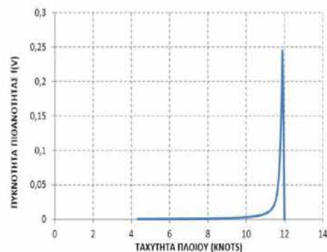
Σχήμα 5.9 Σχηματική μορφή πιθανοτικής κατανομής ταχύτητας πλοίου
