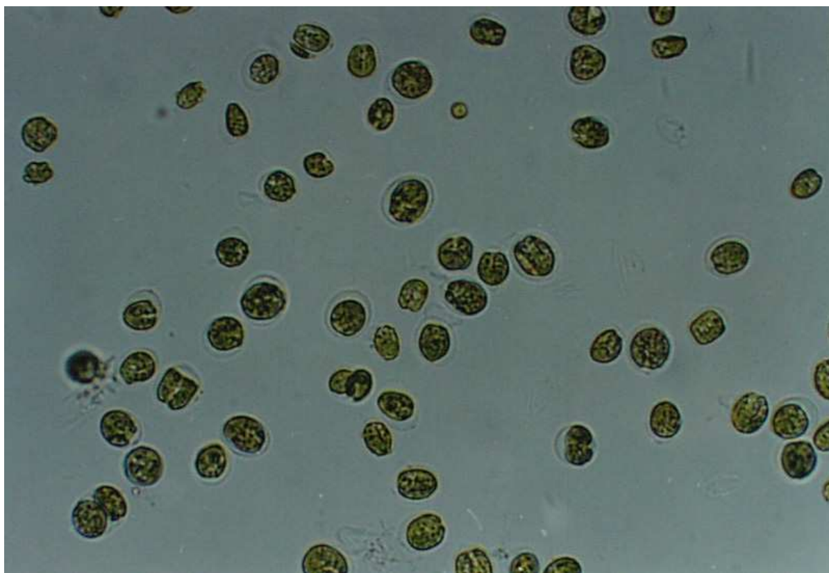
Εικόνα 2. Κύτταρα του γένους Tetraselmis sp.(πηγή: http://www.kmmcc.re.kr/dataroom/product_img/8-25/p02501.jpg ).
