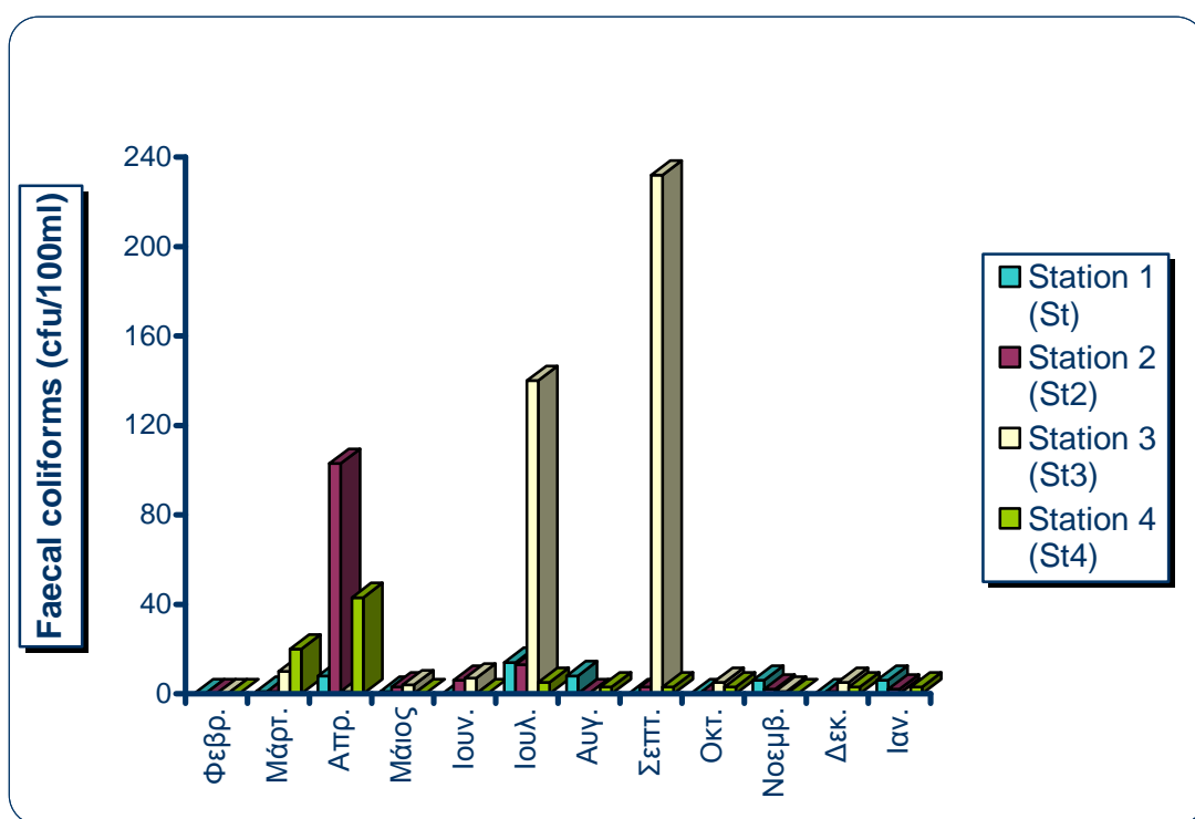
Γράφημα 10. Γράφημα διακύμανσης φορτίου Faecal coliforms
