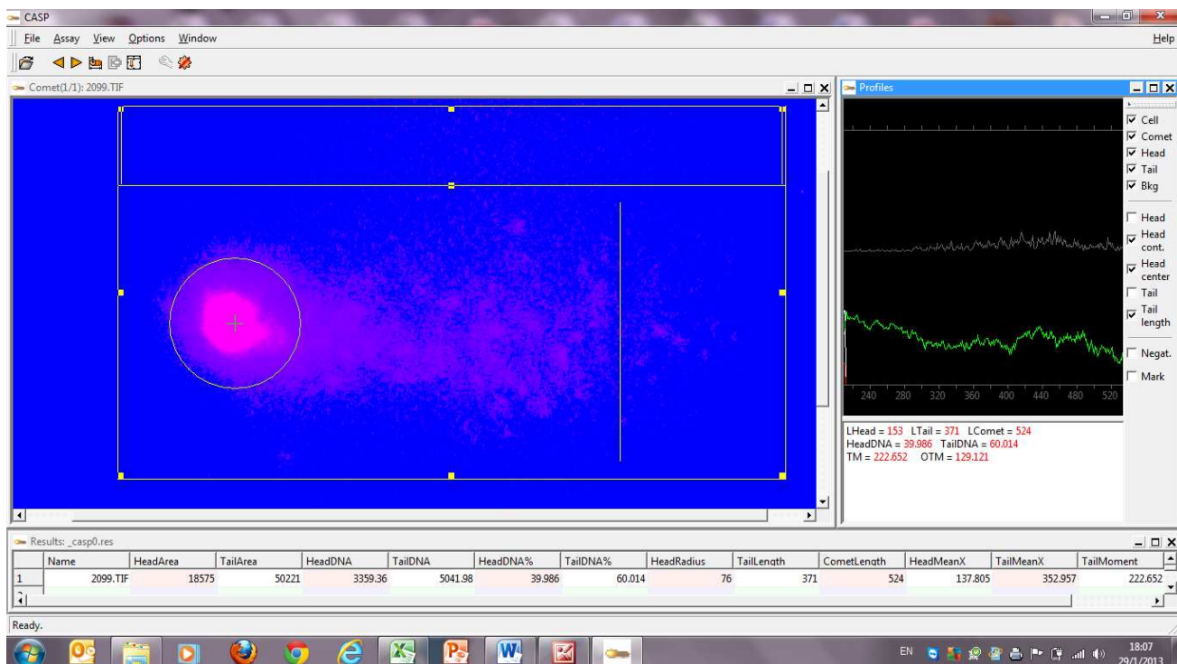
Εικόνα 18: Υπολογισμός των παραμέτρων ( Name, HeadArea, TailArea, HeadDNA, TailDNA, HeadDNA%, TailDNA%, HeadRadius, TailLength, CometLength, HeadMeanX, TailMeanX, TailMoment ) του κατακερματισμού του DNA, μέσω του λογισμικού ανάλυσης εικόνας "casp".
