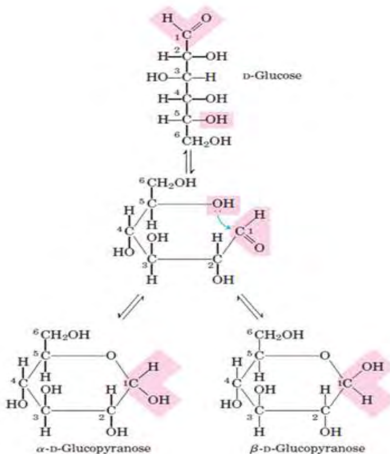
Εικόνα 5. α-D- και β-D- Γλυκοπυρανόζη.
