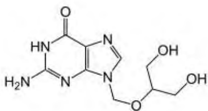
Ganciclovir or DHPG
