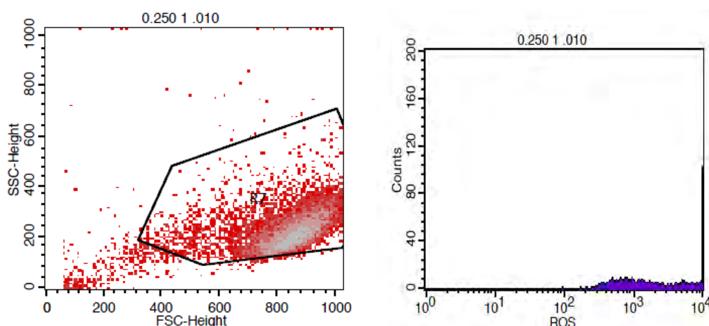
Γράφημα 5: Αντιπροσωπευτικές εικόνες γραφημάτων που δείχνουν την κοκκίωση (SSC) και το μέγεθος (FSC) των κυττάρων EAhy 926 καθώς και τη μεταβολή των ελευθέρων ριζών (ROS) στα κύτταρα EAhy 926. Τα ιστογράμματα δείχνουν τα επίπεδα των ROS μετά από χρώση με DCF υπό φυσιολογικές συνθήκες (control), υπό την επίδραση μόνο του t-BOOH και υπό το συνδυασμό χορήγησης εκχυλίσματος από στέμφυλα και t-BOOH.
