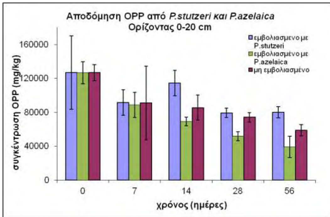
Διάγραμμα 1: Η αποδόμηση του OPP που περιέχεται σε ΕΥΜ από τον ορίζοντα 0-20cm σε υπόστρωμα εμβολιασμένο με P. stutzeri OPP26, υπόστρωμα εμβολιασμένο με P. azelaica PHB-1 καθώς και σε μη εμβολιασμένο ΕΥΜ (Μάρτυρας). Κάθε τιμή αποτελεί το μέσο όρο τριών επαναλήψεων \pm τυπική απόκλιση.
