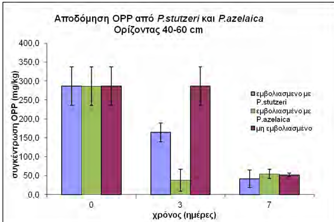
Διάγραμμα 2: Η αποδόμηση του OPP που περιέχεται σε ΕΥΜ που συλλέχθηκε από τον ορίζοντα 40-60cm σε υπόστρωμα εμβολιασμένο με P.stutzeri OPP26, υπόστρωμα εμβολιασμένο με P.azelaica PHB-1, καθώς και σε μη εμβολιασμένο ΕΥΜ (μάρτυρας). Κάθε τιμή αποτελεί το μέσο όρο τριών επαναλήψεων \pm τυπική απόκλιση.
