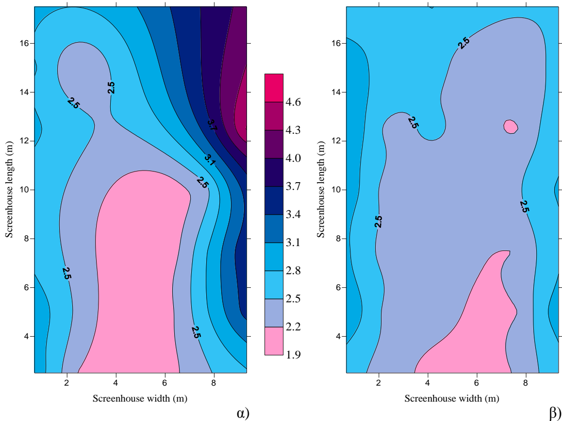
Σχήμα 31. Κατανομή της κανονικοποιημένης μέσης θερμοκρασίας στα διχτοκήπια α)W13 και β) W34.
