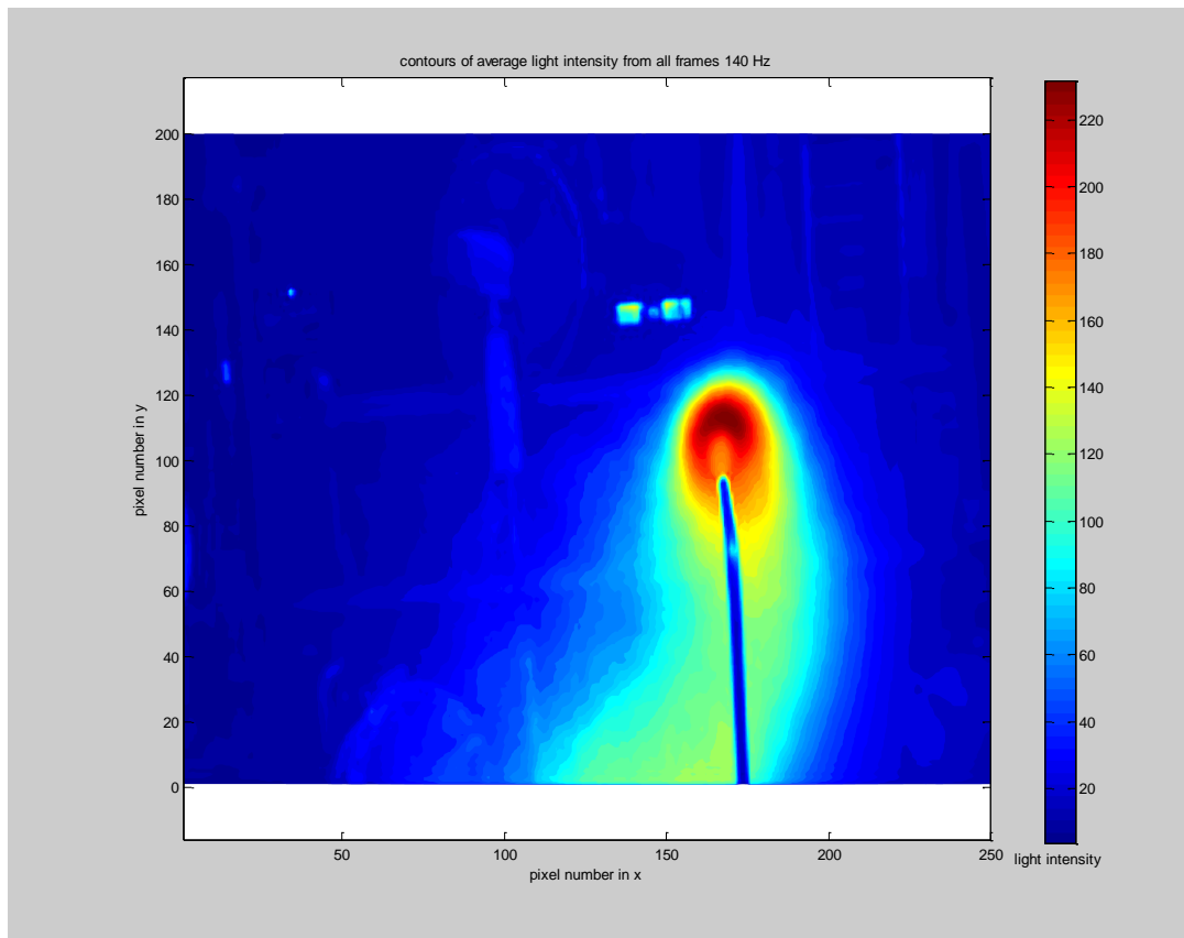
Εικόνα 3.10 140 Hz ισοσταθμικές μέσες καμπύλες συναρτήσεως των pixels μέσω τιμής των frames
