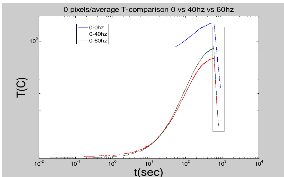
Εικόνα 4.18 η power-40-60Hz θερμοκρασία σε συνάρτηση με το χρόνο σε λογαριθμική κλίμακα για το κέντρο της αντίστασης
