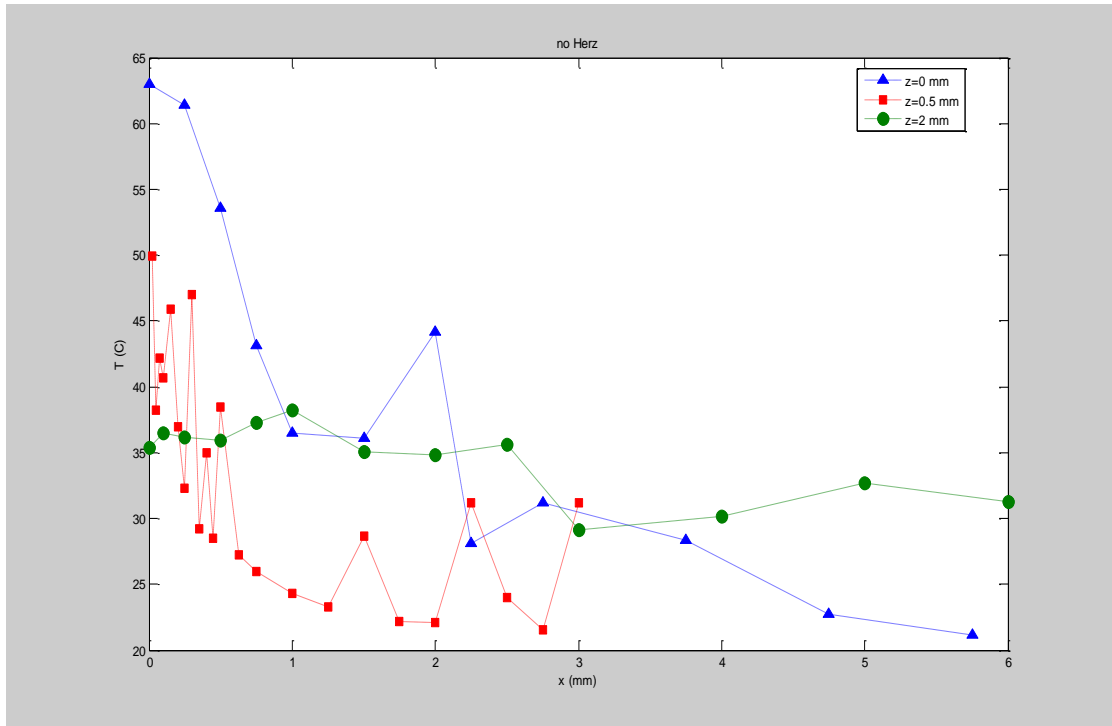
Εικόνα 5.52 no power θερμοκρασία σε συνάρτηση με την εγκάρσια απόσταση x για z=0, 0.5, 2 mm
