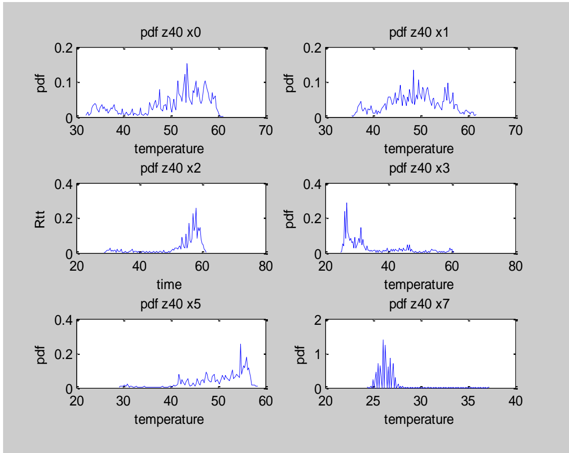
Εικόνα 5.19 P=162 W συνάρτηση πυκνότητας πιθανότητας (pdf) για ύψος z=40 mm
