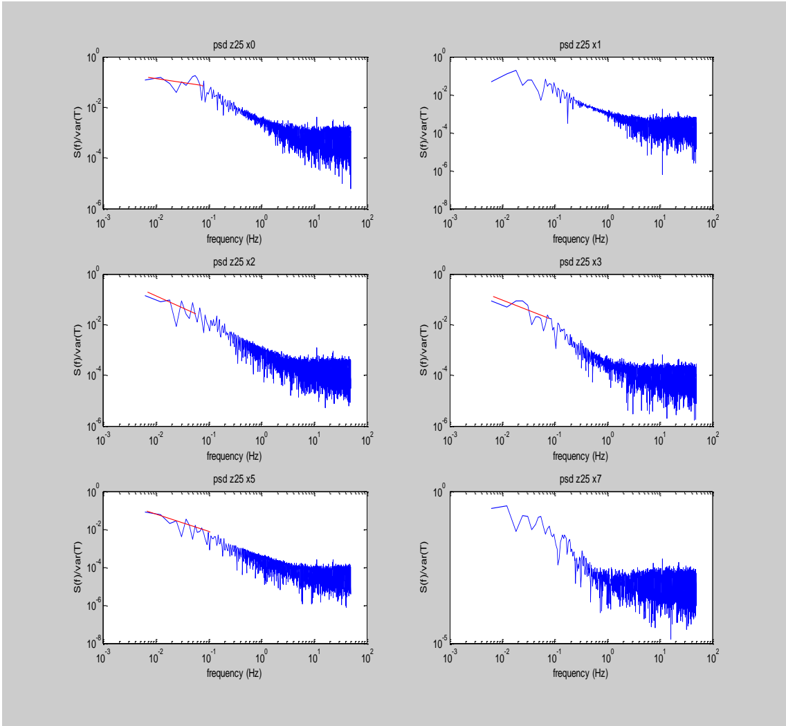
Εικόνα 5.38 P=162\text{ W} power spectral density (psd) για ύψος z=25\text{ mm}
