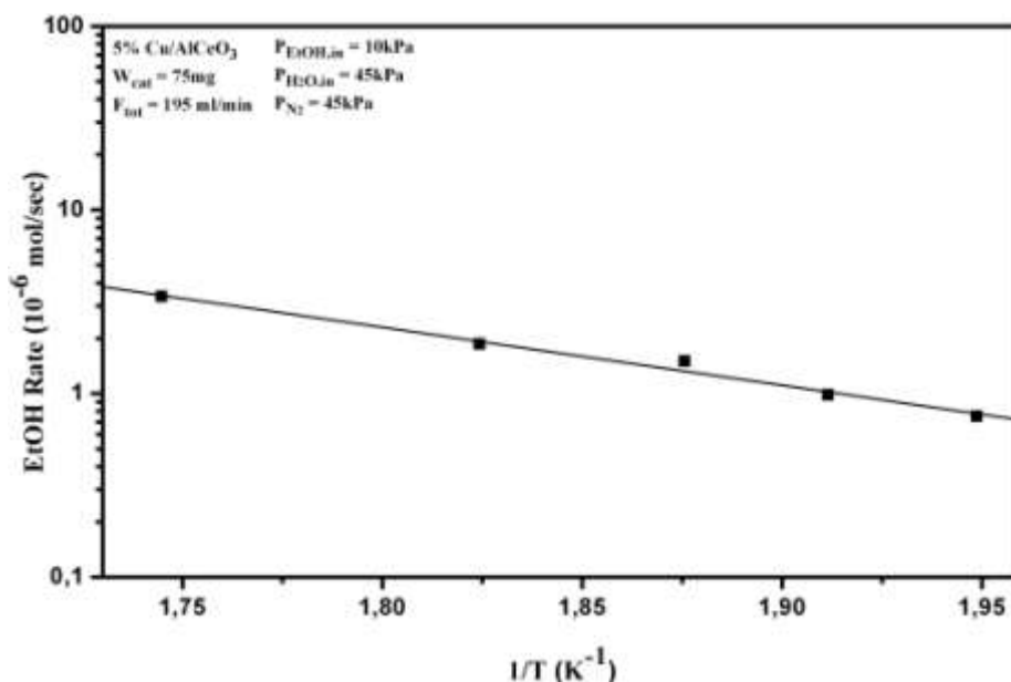
Σχήμα 5.32: Διάγραμμα Arrhenius του ρυθμού μετατροπής της αιθανόλης κατά την αντίδραση αναμόρφωσης με ατμό, σε φορέα 5%wt.Cu/AlCeO 3 . P_{\text{tot}}=1\text{atm} , παροχή υγρού μίγματος 0.1 ml/min, συνολική παροχή στην αέρια φάση 195 cm 3 /min.
