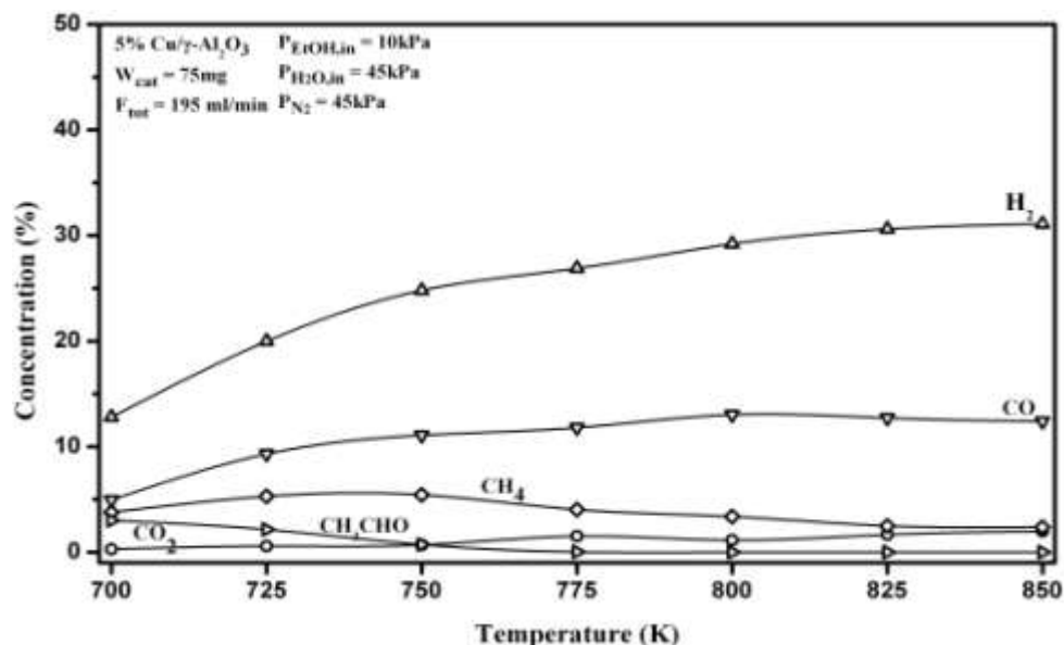
Σχήμα 5.19: Επίδραση της θερμοκρασίας στις συγκεντρώσεις των CO, CO 2 , H 2 , Ac και CH 4 κατά την αντίδραση αναμόρφωσης με αιμό, σε καταλύτη 5 wt.% Cu/γ-Al 2 O 3 . P tot =1atm, παροχή υγρού μίγματος 0.1 ml/min, συνολική παροχή στην αέρια φάση 195 cm 3 /min.
