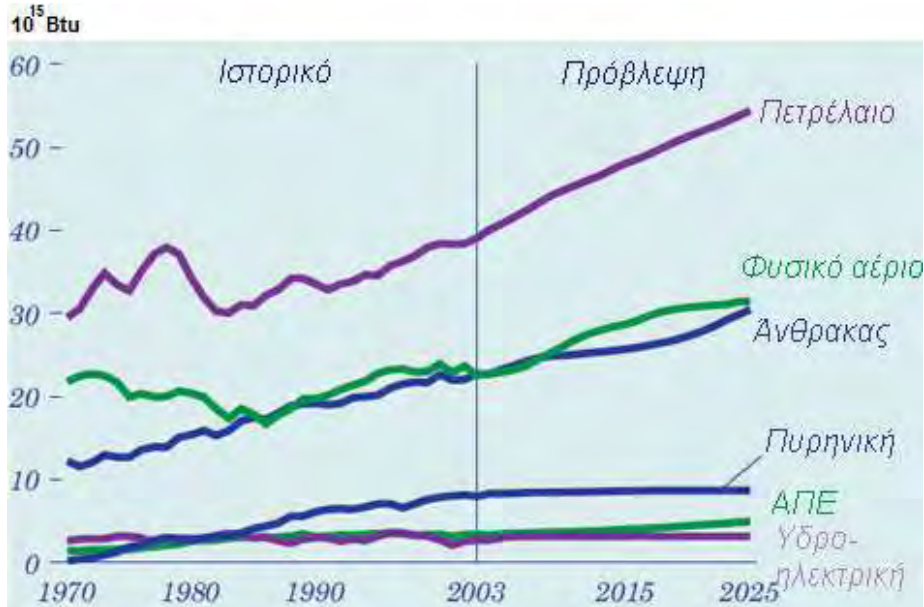
Σχήμα 1.3: Κατανάλωση ενέργειας ανά τύπο καυσίμου [1,2]
