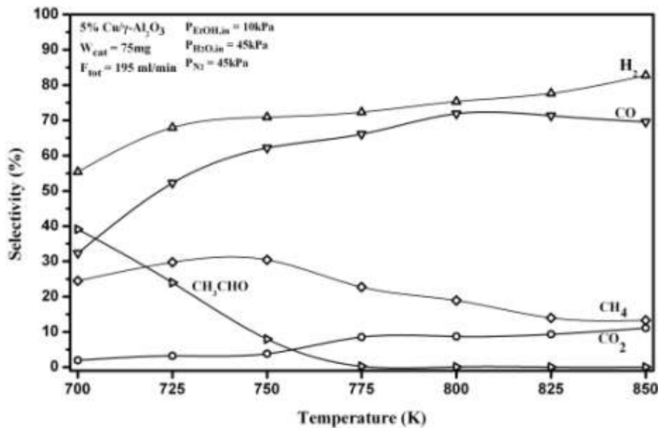
Σχήμα 5.18: Επίδραση της θερμοκρασίας στις εκλεκτικότητες των CO, CO 2 , H 2 , Ac και CH 4 κατά την αντίδραση αναμόρφωσης με αιμό, σε καταλύτη 5 wt.% Cu/γ-Al 2 O 3 . P tot =1atm, παροχή υγρού μίγματος 0.1 ml/min, συνολική παροχή στην αέρια φάση 195 cm 3 /min.
