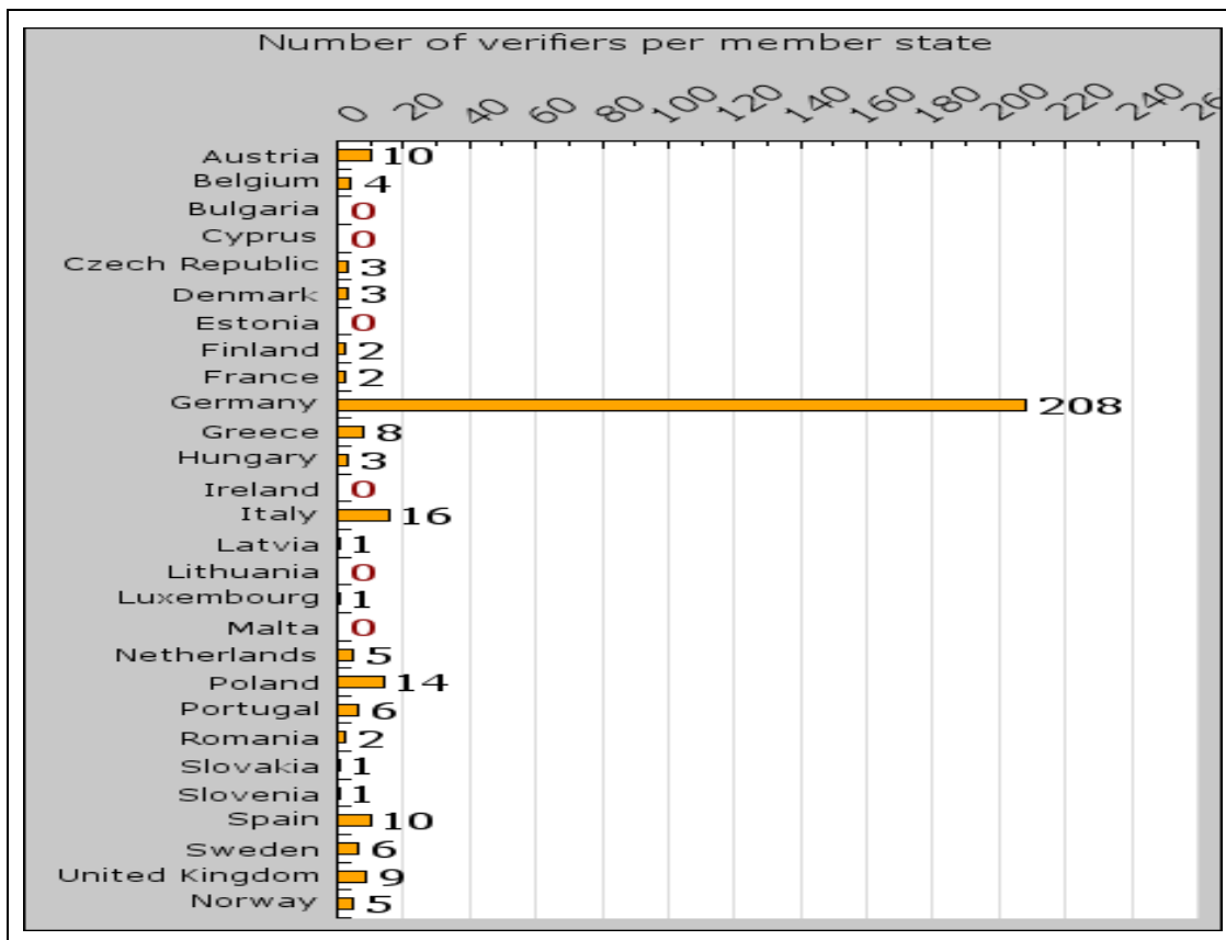
Σχήμα 3.2 : Διαπιστευμένοι Επαληθευτές Περιβάλλοντος EMAS στον ευρωπαϊκό χώρο (10/06/2010)
