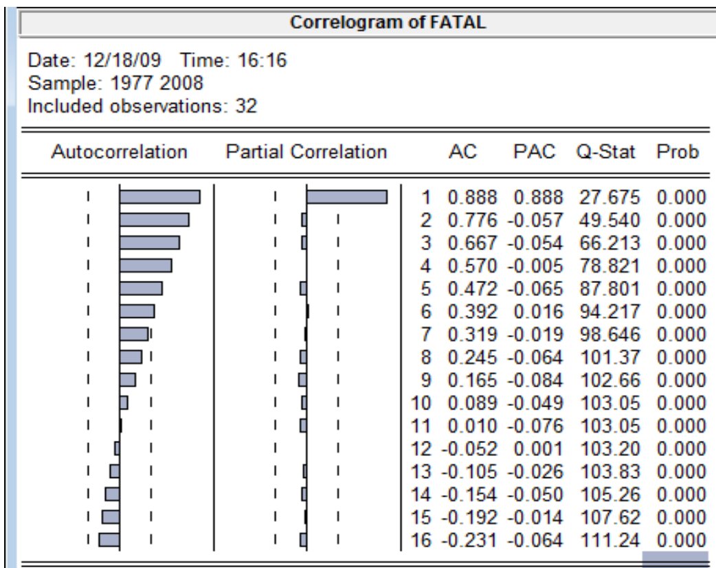
Συνάρτηση Αυτοσυσχέτισης και Μερικής Αυτοσυσχέτισης (fatal accidents)
