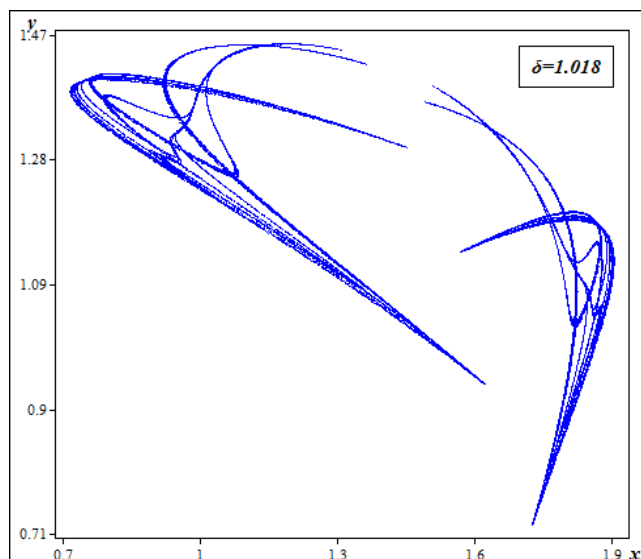
Σχήμα 6.15(ε) Διάγραμμα φάσεων για \delta = 1,018
