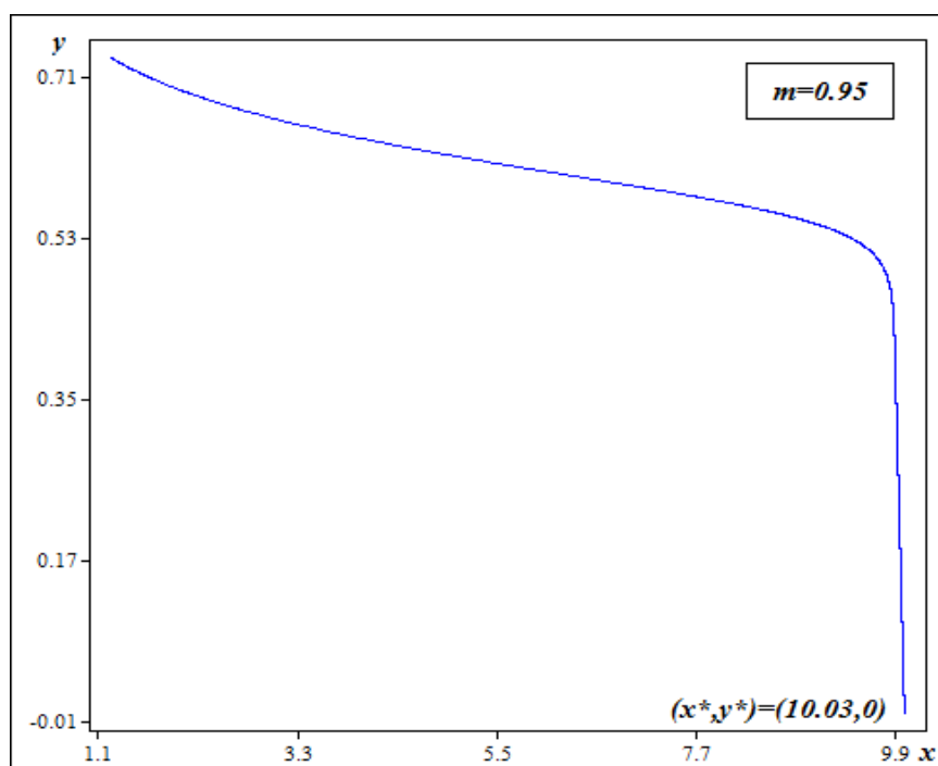
Σχήμα 7.5 Διάγραμμα φάσεων για 0,9 < m < 1
