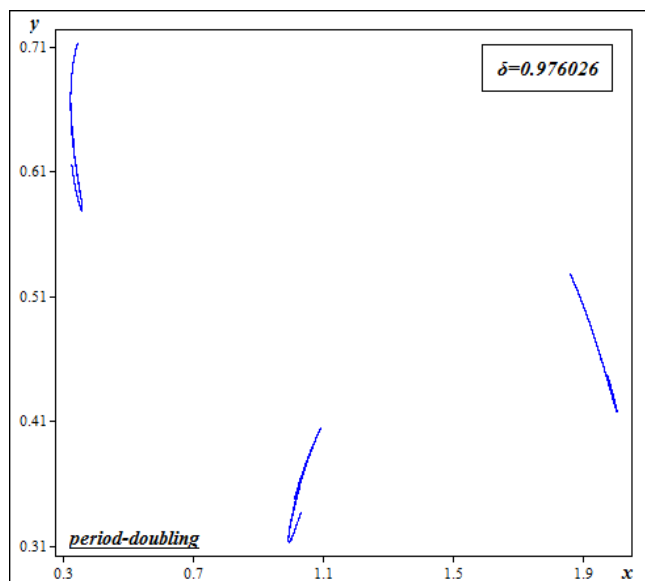
Σχήμα 6.5(α) Διάγραμμα φάσεων για \delta = 0,976026
