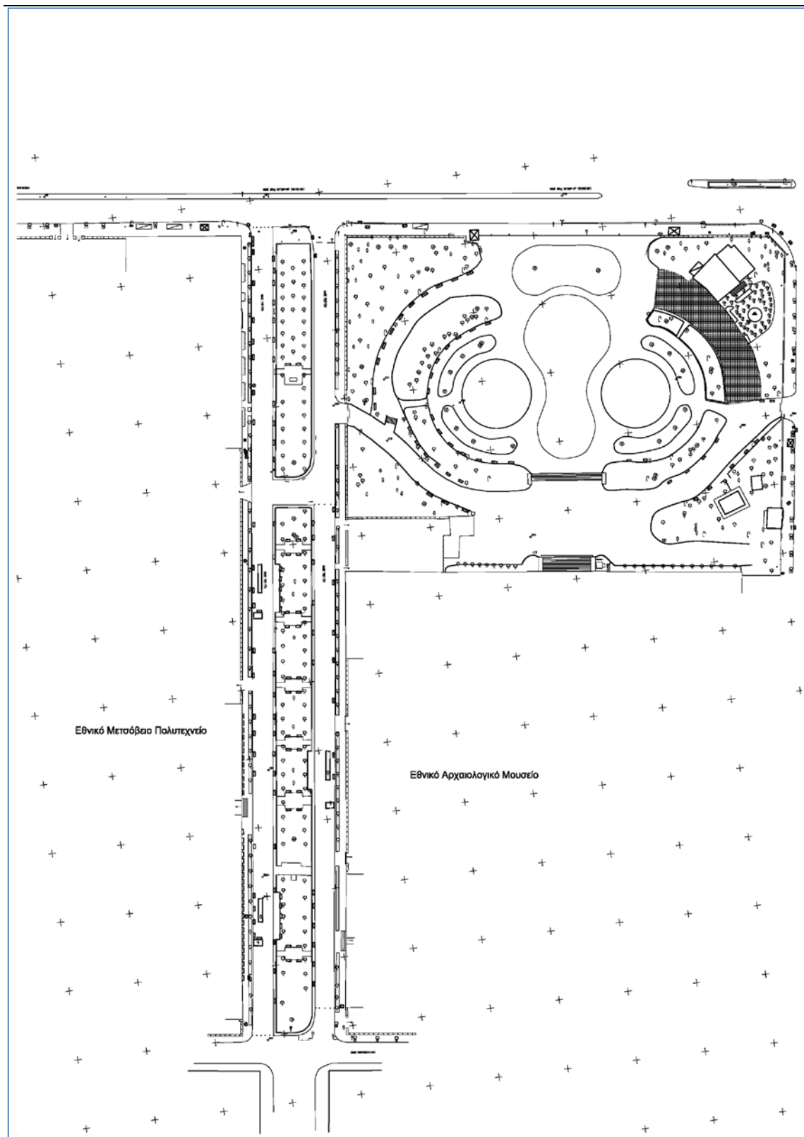
Τοπογραφική αποτύπωση οδού Τσιτσά
