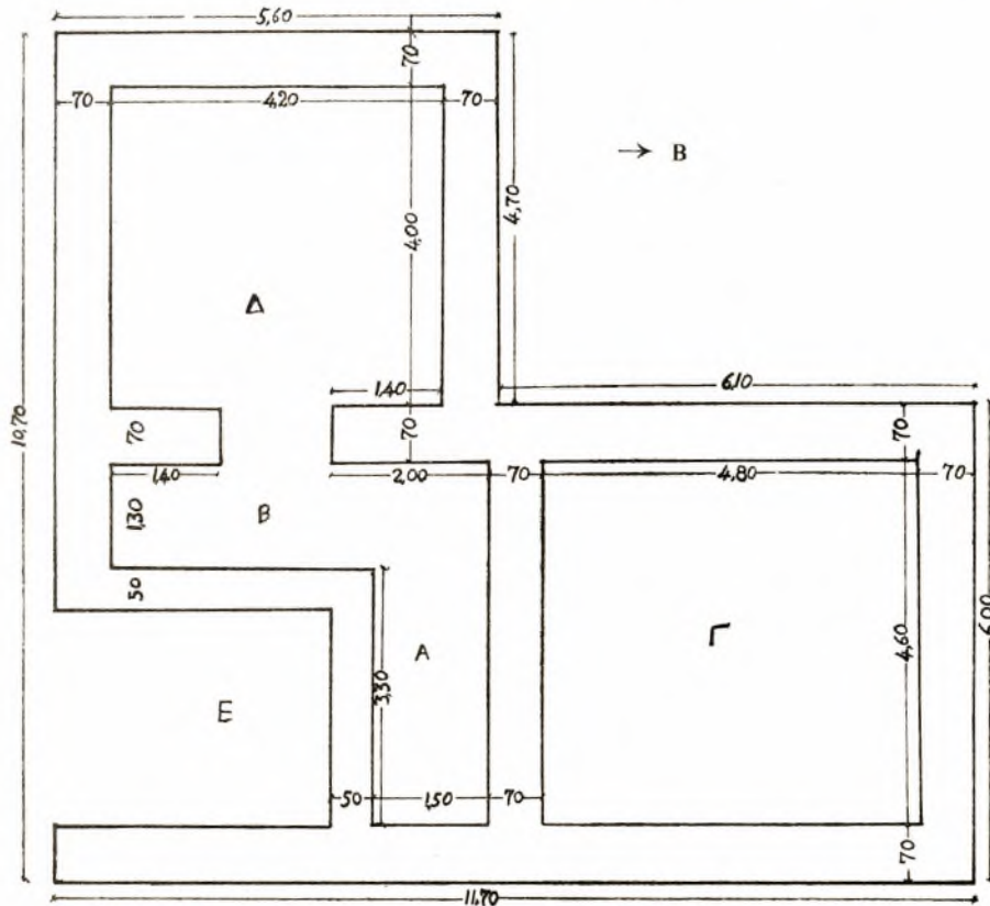
Σχ ἐ δ. 1. Κάτωγες Ρωμαϊκῆς ἐπαύλεως, ἀποκαλυφθείσης εἰς οἰκόπεδον Παρασκευοπούλου εἰς Σπάρτην
