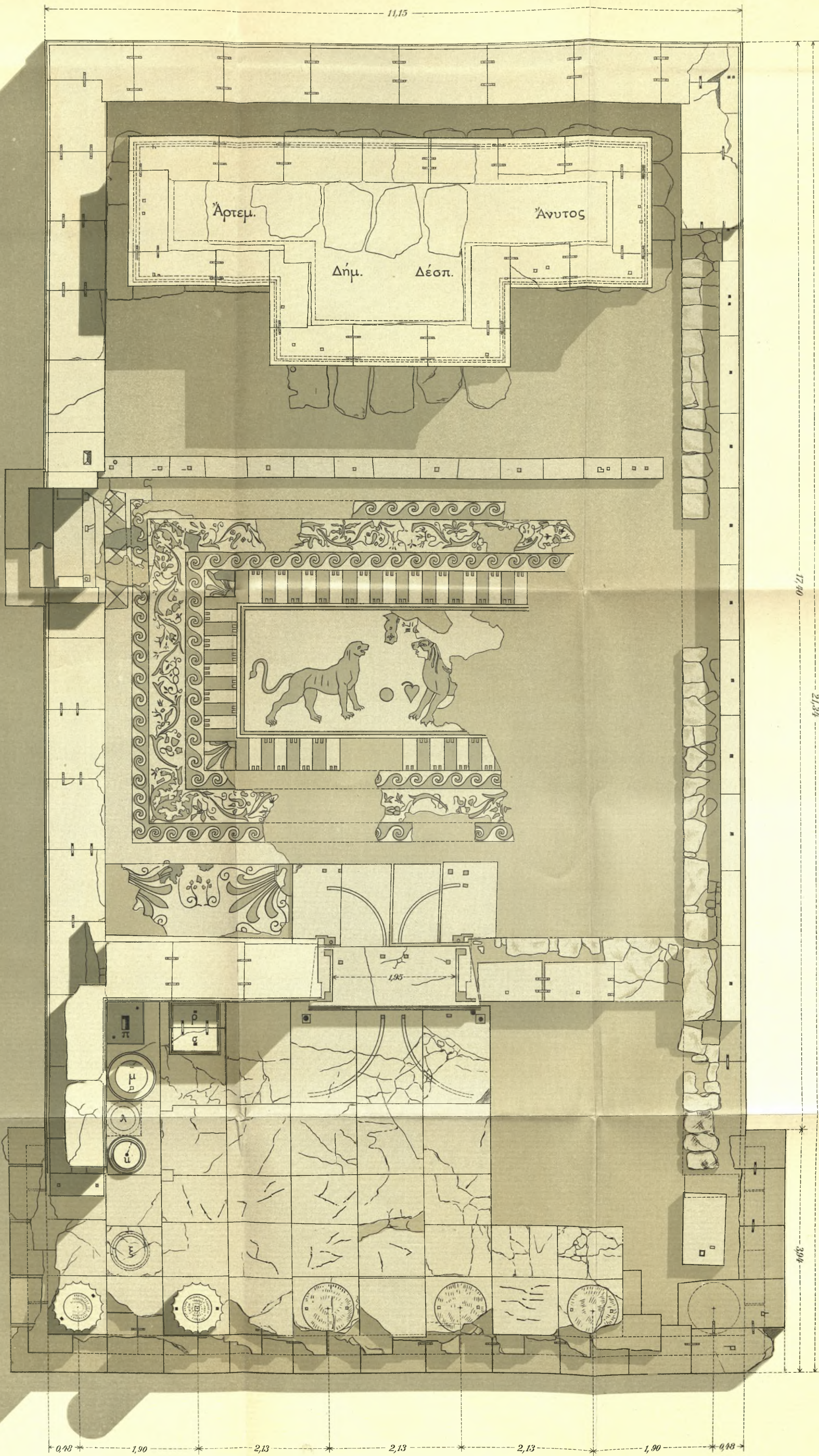
ΚΑΤΟΨΙΣ ΤΟΥ ΕΝ ΛΥΚΟΣΟΥΡΑΙ ΝΑΟΥ ΤΗΣ ΔΕΣΠΟΙΝΗΣ
