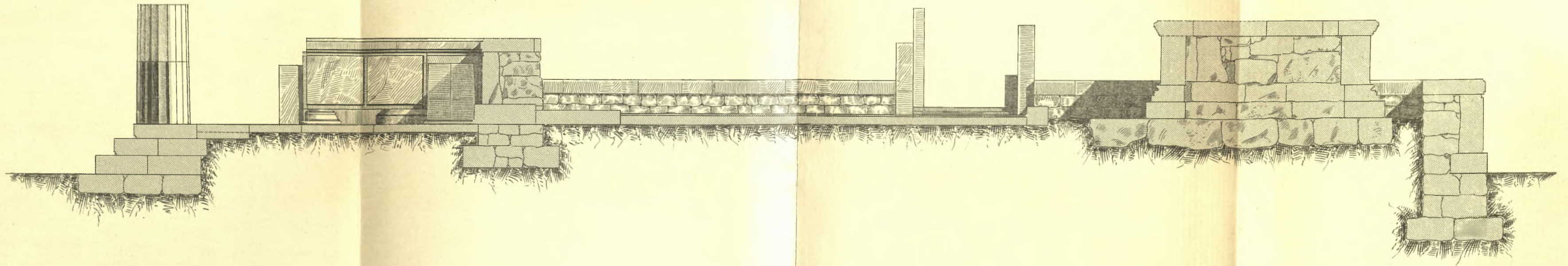
(Α) ΚΑΤΑ ΜΗΚΟΣ ΤΟΜΗ ΤΟΥ ΕΝ ΛΥΚΟΣΟΥΡΑΙ ΝΑΟΥ ΤΗΣ ΔΕΣΠΟΙΝΗΣ
