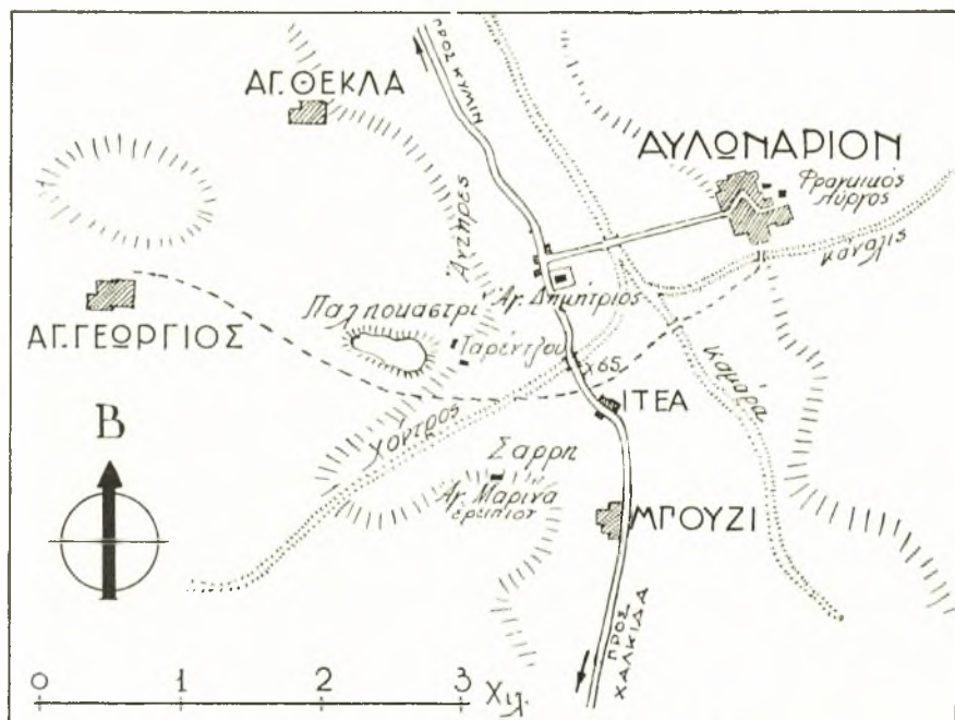
Εικ. 2. Τοπογραφικόν διάγραμμα τής περιοχής του Αύλωναρίου.
