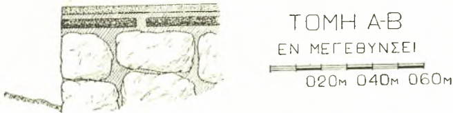
Εἰκ. 3 γ. Τμήμα ῥωμαϊκοῦ κτίσματος.
