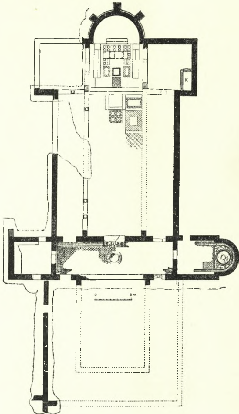
Σχεδ. 1. Κάτωρις τῆς Βασιλικῆς Δ τῆς Νικοπόλεως
