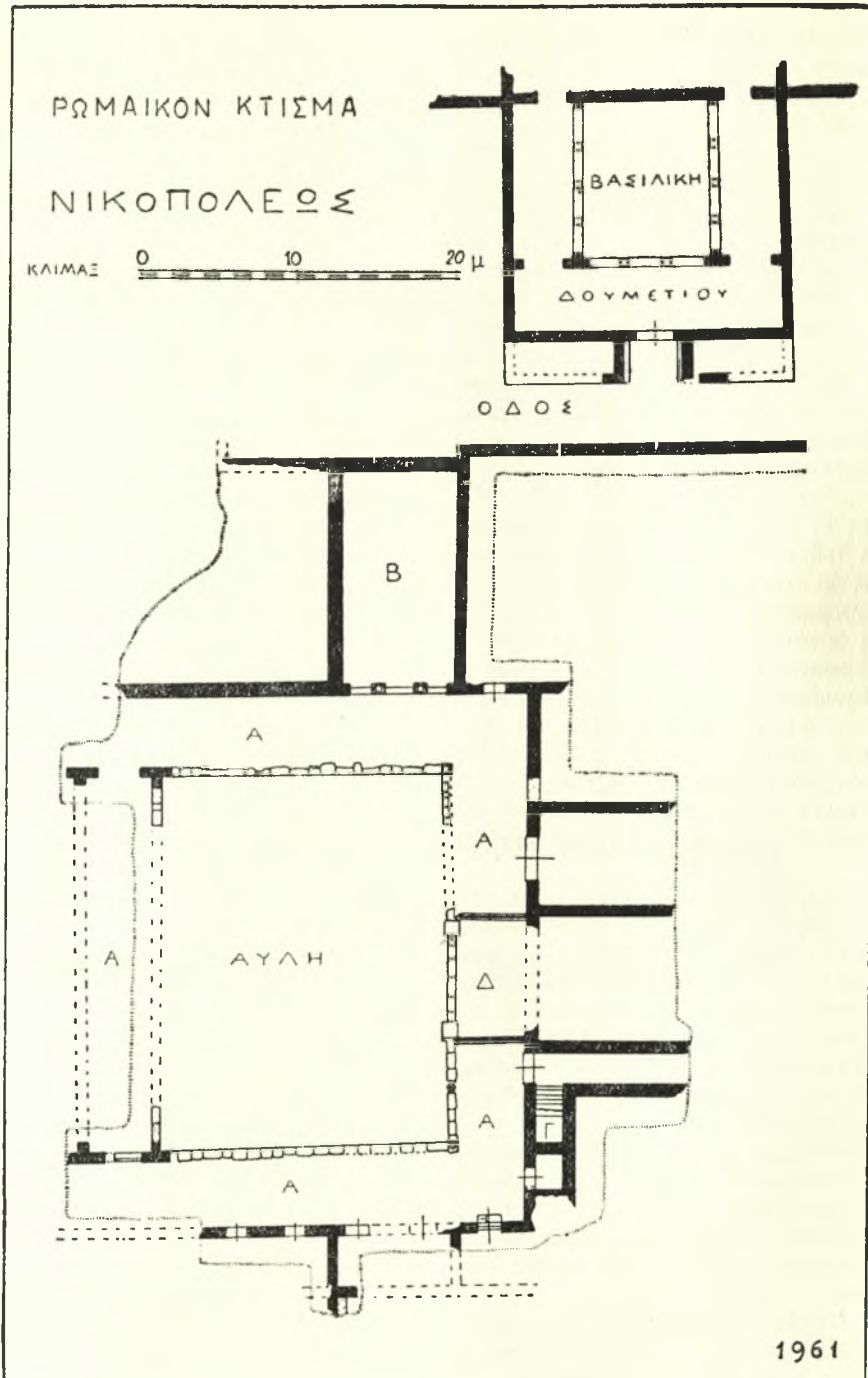
Σχεδ. 2. Κάτωφισ τοῦ δυτικῶς τῆς βασιλικῆς τοῦ Δουμετίου ρωμαϊκοῦ κτηρίου, χρησιμοποιηθέντος πιθανῶς ἀργότερον ὡς ἐπισκοπικοῦ μεγάρου
