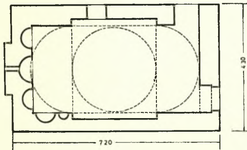
Σχέδ. 3. Ναός Παναγίας τοῦ Βουνοῦ. Βορεῖα ὄψεις καὶ κάτοψις
