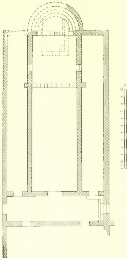
Εἰκ. 2. Σχέδιον τῆς παλαιοχριστιανικῆς βασιλικῆς εἰς θέσιν Κερά 'Ονουθῆ Γουλεδιανῶν.
