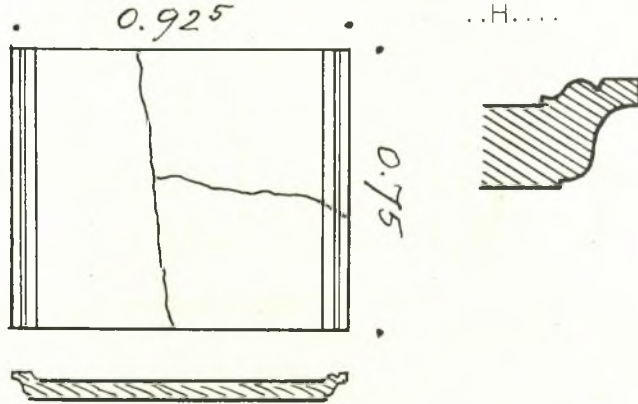
Εἰκ. 7. Τμήμα καλυπτηρίου πλακῶς Ἄγ. Τραπέζης μετ' ἀνασκαμμένων χειλῶν.
