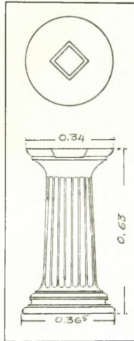
Εἰκ. 10. Βάσις λεκάνης ἀρχαίου περιρραντηρίου στηρίζουσα τὴν λεκάνην ἁγιασμοῦ.
