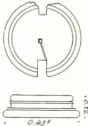
Εἰκ. 6. Ἴωνικὴ βᾶσις κίονος.
