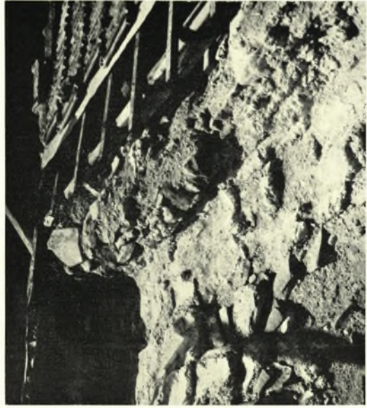
Φθιώτις, Μονή Ἀγίου: α. Ἀνατολική ὄψις πρὸς τῆς ἀφαιρέσεως τῶν κονιαμάτων, β. Ὁ ἀποκαλυφθεὶς τρουλλίσκος τοῦ παρεκκλησίου τῆς Μεταμορφώσεως πρὸ τῶν ἐργασιῶν, γ. Ἡ στέγη τοῦ παρεκκλησίου τῆς Μεταμορφώσεως πρὸ τῶν ἐργασιῶν, δ. Ἡ παλαιὰ καὶ ἡ νέα στέγη
