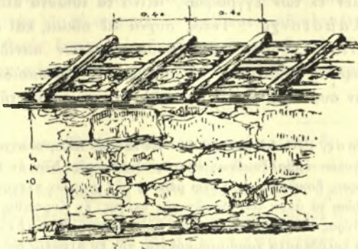
Εἰκ. 2. Πῶς γίνεται τὸ ξυλόδεμα νῦν ἐν Αἰτωλίᾳ. (Δ. Λουκοπούλου, Αἰτωλικαὶ οἰκῆσεις σ. 42).
