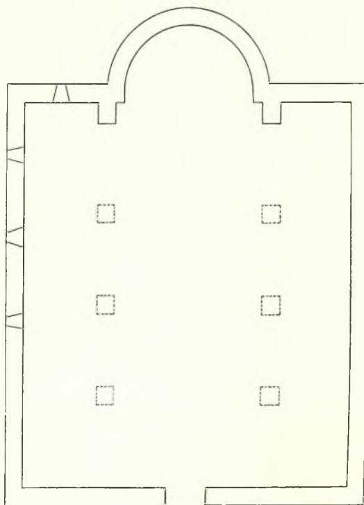
Σχέδ. 3. Σκίαθος. Ναὸς Ἁγίας Τριάδος. Κάτωψις
