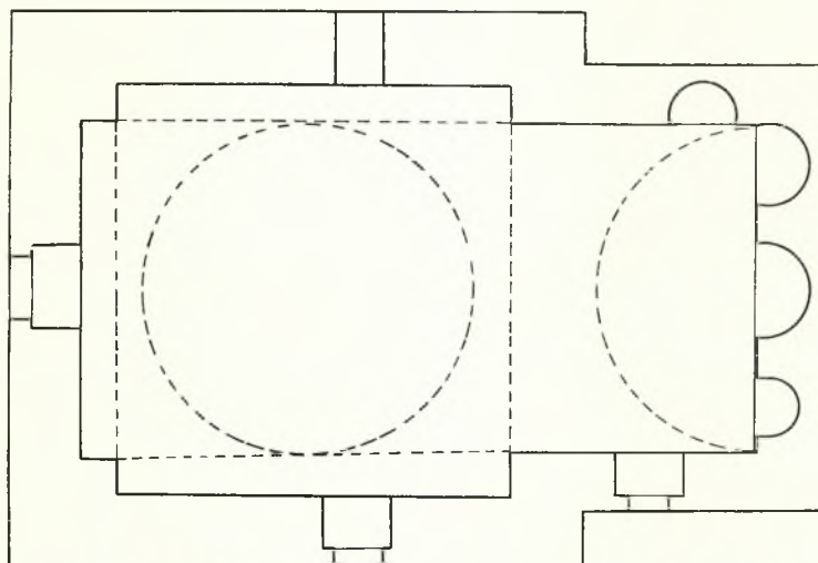
Σχέδ. 4. Σκίαθος. Μονὴ Ἁγίου Χαραλάμους. Κάτωφιν Καθολικοῦ
