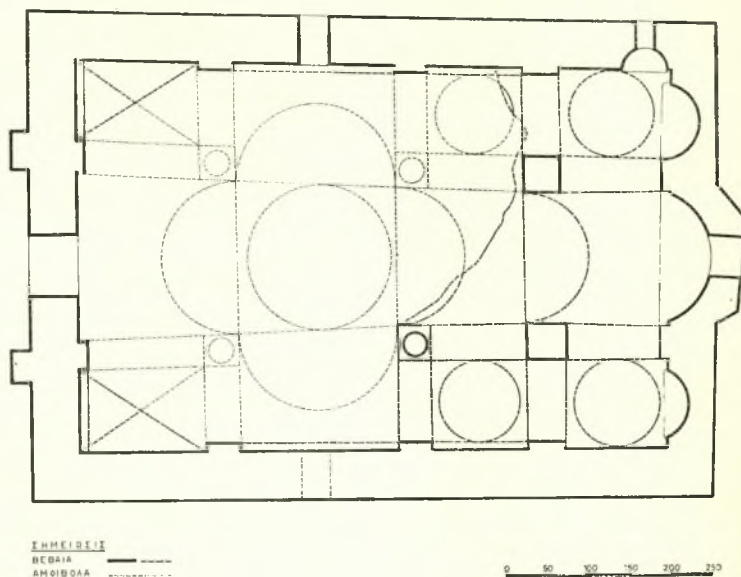
Σχέδ. 8. Σκιάθος. Βυζαντινὸς ναὸς Ἐθαγγελισμοῦ. Κάτωψις
