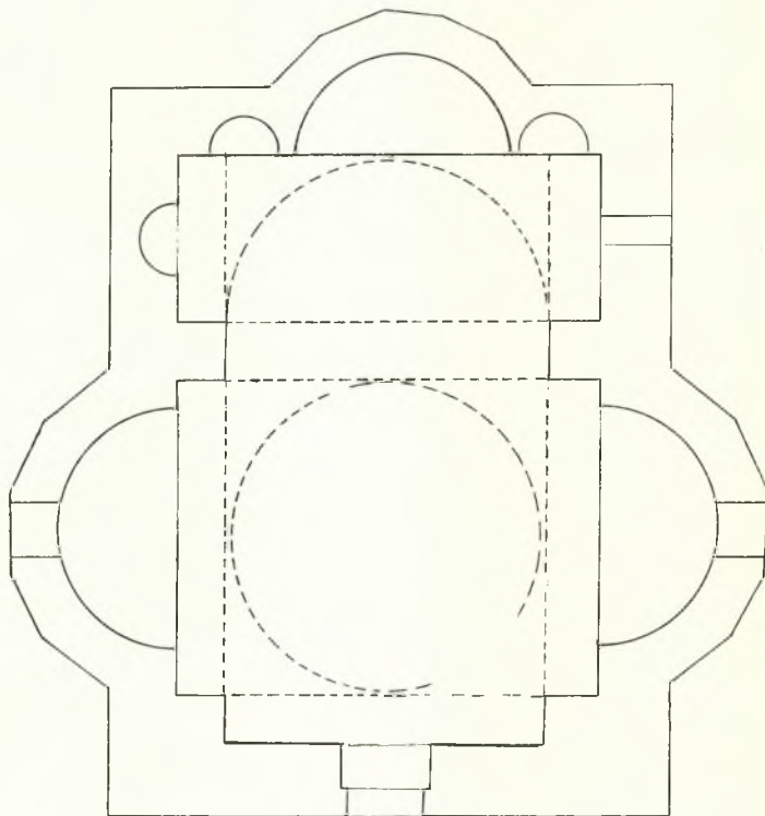
Σχέδ. 6. Σκιάθος. Καθολικὸν μονῆς Κεχρεῶς. Κάτοπις
