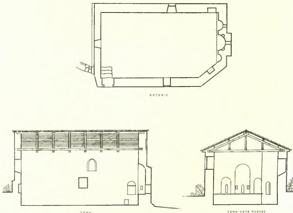
Σχέδ. 5. Σκιάθος. Κάτοπις καὶ τομαὶ τοῦ «Χριστοῦ στὸ Κάστρο»
