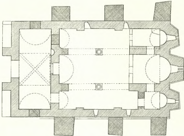
Σχέδ. 4. Καμένα Βοῦρλα. Μονὴ Μεταμορφώσεως ἢ Ἁγιά. Κάτωψις
