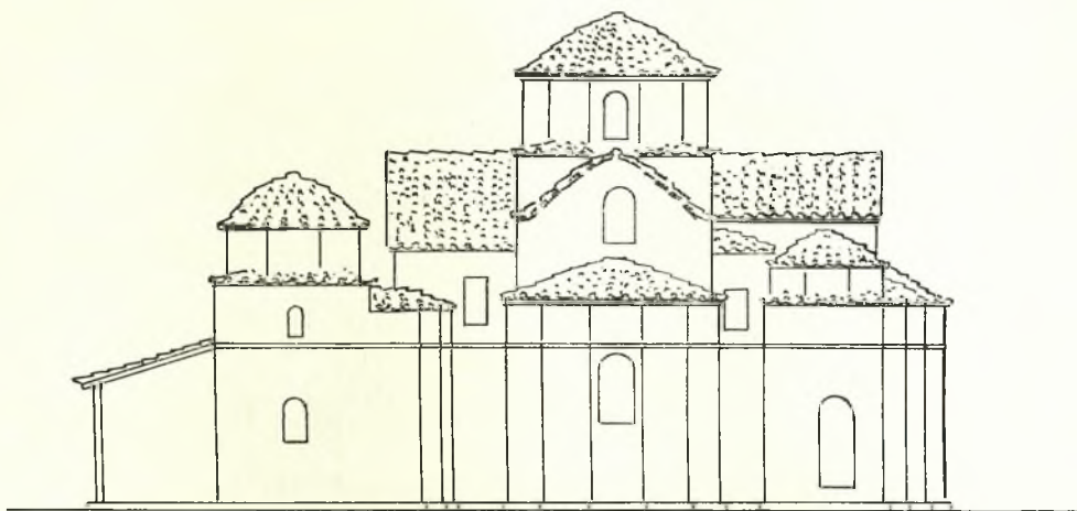
Σχέδ. 2. Καθολικὸν Μονῆς Ἀγάθωνος. Νοτία ὄψεις μετὰ τὰς ἐργασίας
