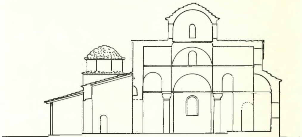
Σχέδ. 1. Κατὰ μῆκος τομὴ Καθολικοῦ Μονῆς Ἀγάθωνος
