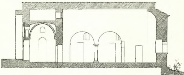
Σχέδ. 5. Καμένα Βοῦρλα. Μονὴ Μεταμορφώσεως ἢ Ἁγιά. Κατὰ μῆκος τομὴ
