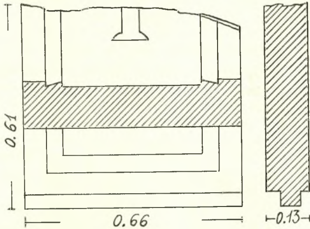
Εἰκ. 4. Πῶρινον θωράκιον. Ὅψις καὶ τομαί.
