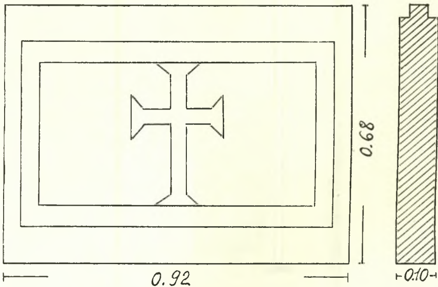
Εἰκ. 3. Πύρινον θωράκιον. Ὅψις καὶ τομή.
