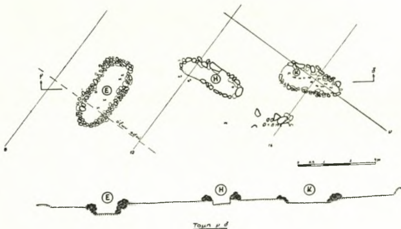
Σχεδ. 6. Τομὴ γ-δ τοῦ τύμβου III
