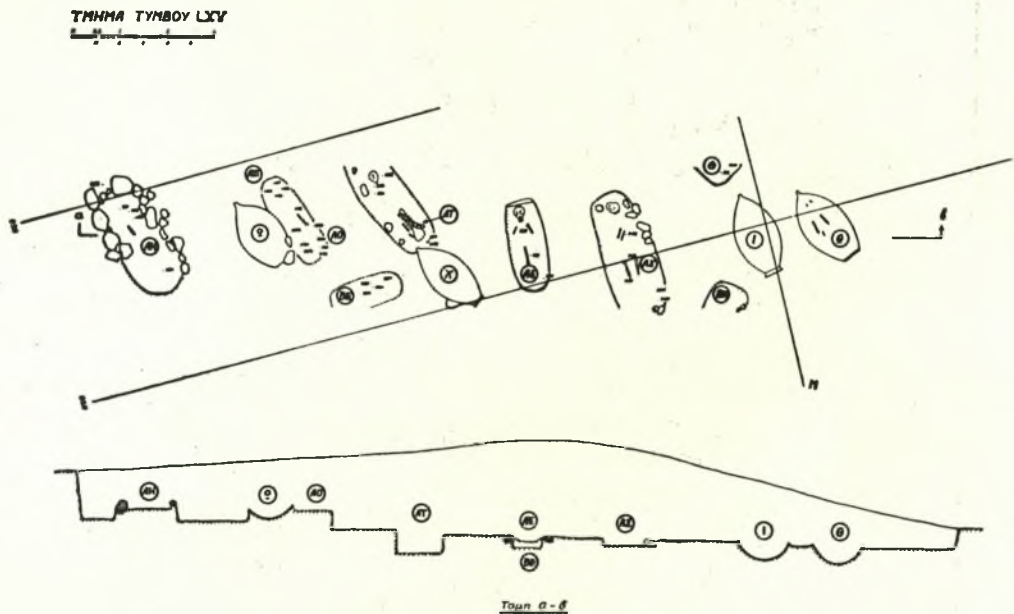
Σχεδ. 48. Τομή α-β τοῦ τύμβου LXV
