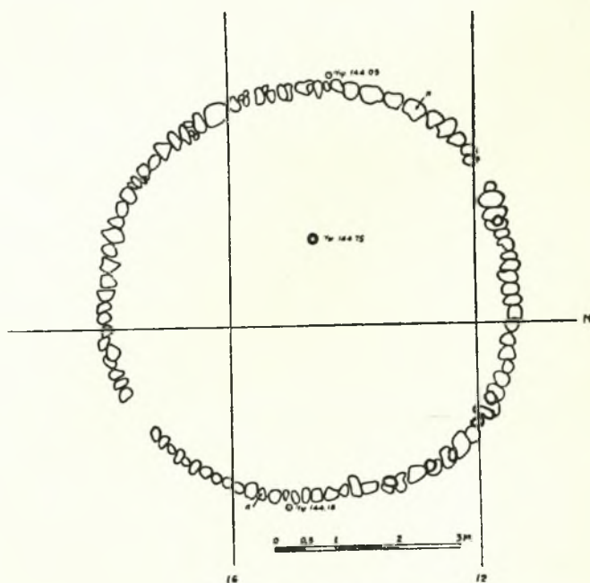
Σχ.δ. 19. Ὁ τύμβος XII
