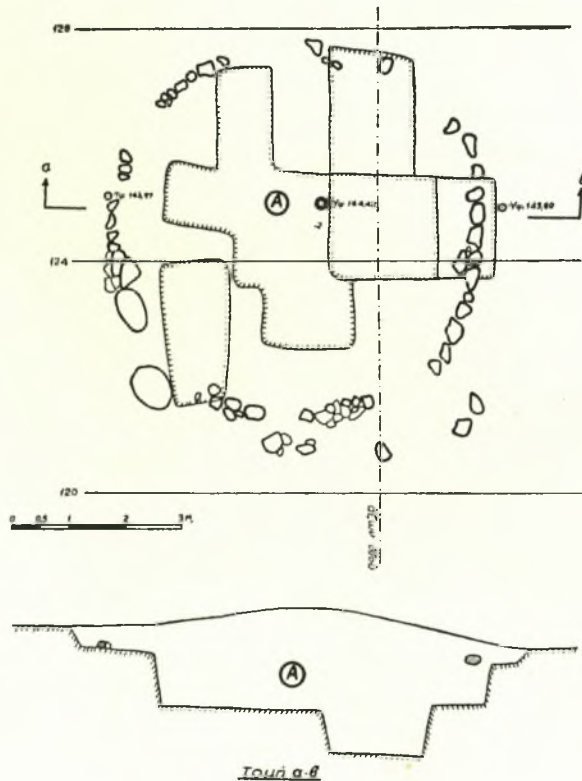
Σχεδ. 38. Ό τύμβος XXXVIII, κάτοψις και τομή α-β
