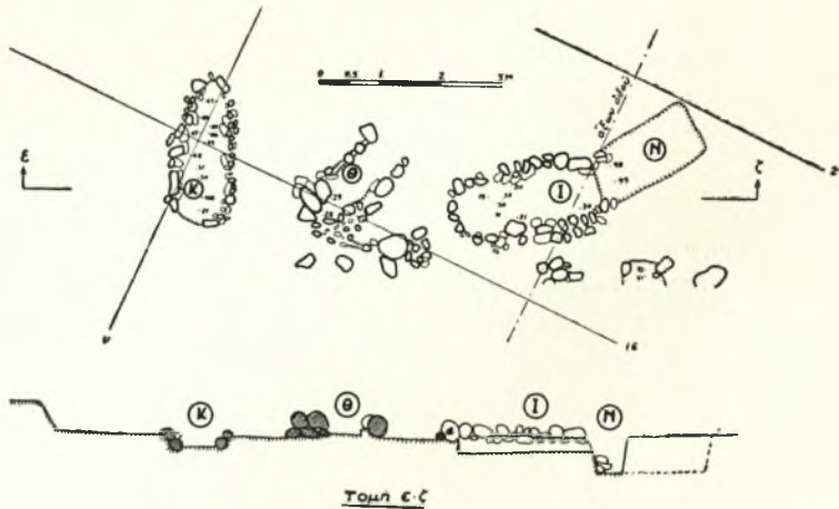
Σχέδ. 7. Τομή ε-ζ τοῦ τύμβου ΙΙΙ
