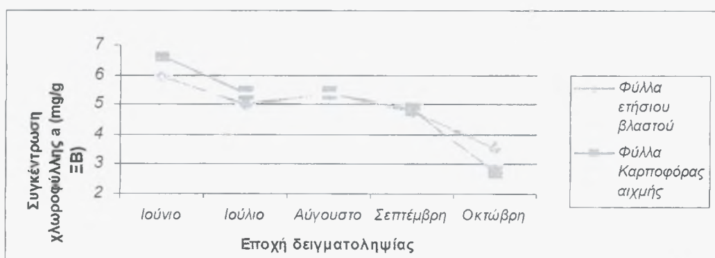
Σχήμα 3.2 Μεταβολή της συγκέντρωσης της χλωροφύλλης a σε σχέση με το χρόνο σε φύλλα ετήσιων βλαστών και καρποφόρων αιχμών σε μηλιές του σπωρώνα του Δ Θλιβερού.
