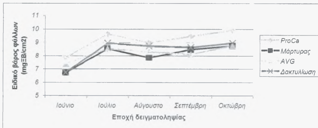
Σχήμα 3.11 Μεταβολή Ειδικού Βάρους Φύλλων σε σχέση με το χρόνο στις τέσσερις μεταχειρίσεις σε φύλλα μηλιάς του οπωρώνα του Δ Θλιβερού .
