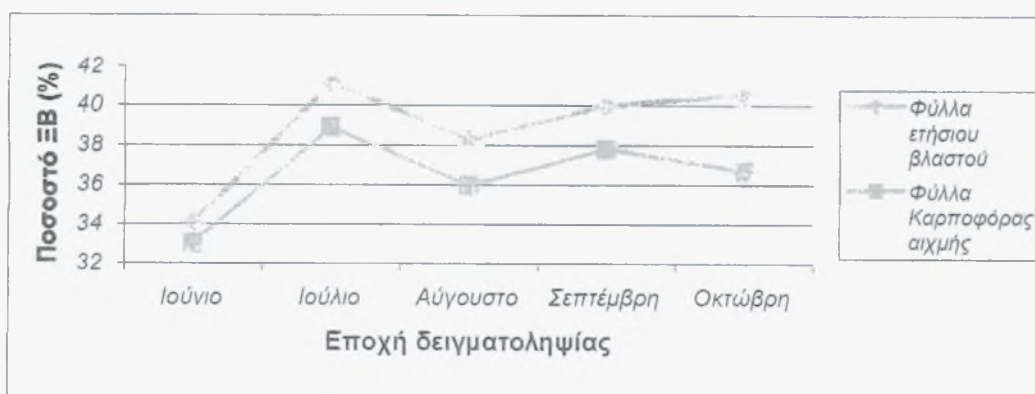
Σχήμα 3.10 Μεταβολή του %ποσοστού ΞΒ σε σχέση με το χρόνο σε φύλλα ετήσιων βλαστών και καρποφόρων αιχμών σε μηλιές του σπρωάνα του Δ Θλιβερού.
