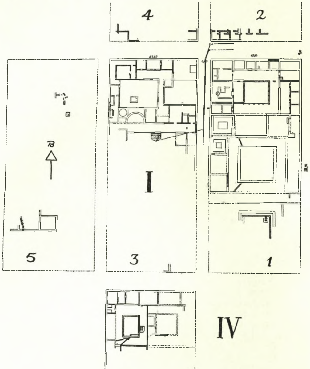
Σχέδ. 1. Κάτοπις τῶν τομέων I καὶ IV
