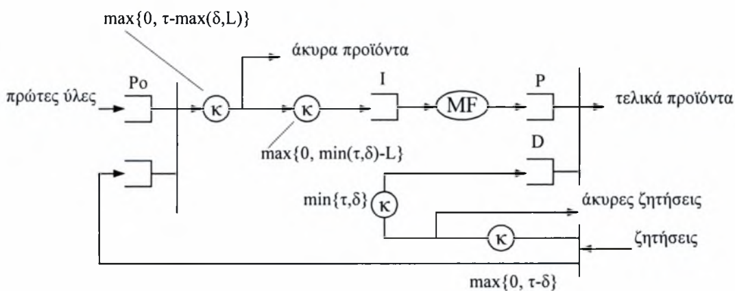
Σχήμα 5.1.1 : Σύστημα με προθεσμία επιβεβαίωσης της ζήτησης και καθυστέρηση
