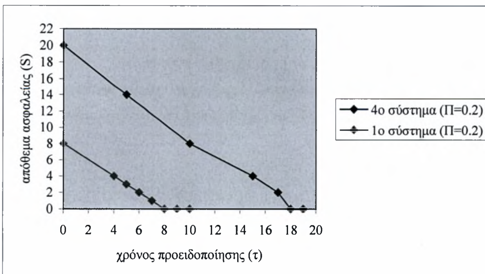
Διάγραμμα 5.1.14 : Συγκριτικά το πρώτο και το τέταρτο σύστημα για \Pi=0.2
