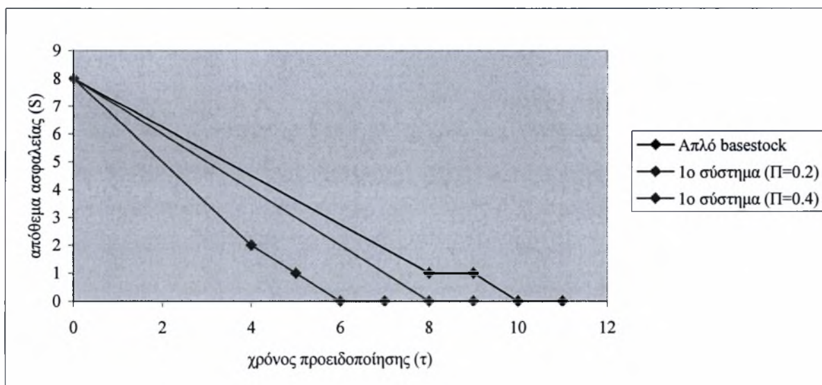
Διάγραμμα 5.1.4 : Συγκριτικά το S^* συναρτήσει του \tau
