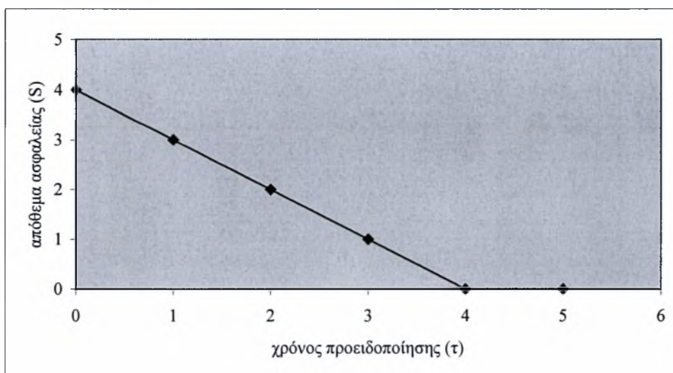
Διάγραμμα 5.1.9 : Το S^* συναρτήσει του \tau για το τρίτο σύστημα και \Pi=0.2
