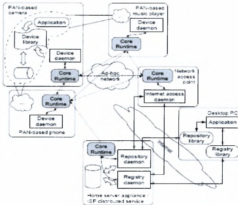
Σχήμα 1.1: Αρχιτεκτονική OmniStore
