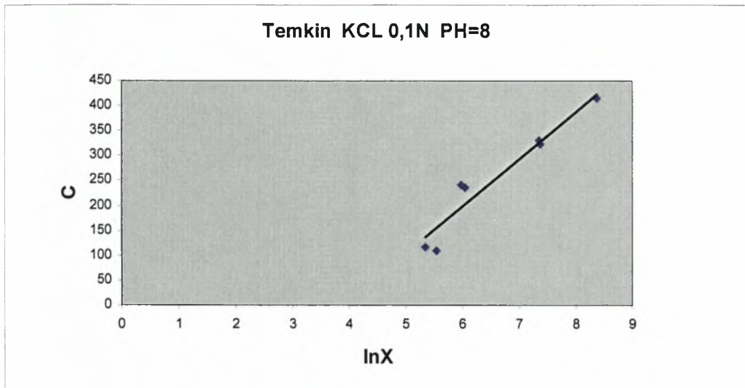
Διάγραμμα 3.4-5: Η συγκέντρωση ισορροπίας C (µg Cd/40ml) σε συνάρτηση με την ln του ποσού που προσροφάται σε pH=8 και παρουσία ηλεκτρολύτη KCl=0,1N.
