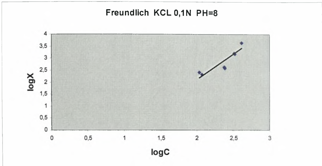
Διάγραμμα 3.3-5: Ο λογάριθμος του ποσού που προσροφάται σε συνάρτηση με τον λογάριθμο της συγκέντρωσης ισορροπίας σε pH=8 και παρουσία ηλεκτρολύτη KCl=0,1N.
