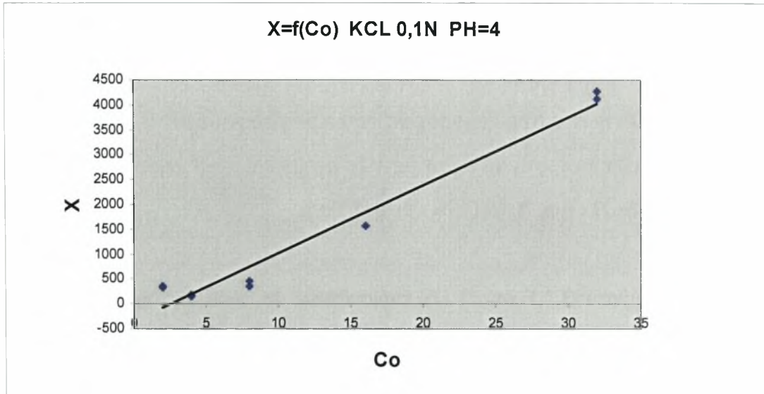
Διάγραμμα 3.1-1: Η προσρόφηση του καδμίου X (μg Cd/g γκαιτίτη) σε συνάρτηση με την αρχική συγκέντρωση του καδμίου Co (μg Cd/ml διαλύματος) σε pH=4 και ηλεκτρολύτη KCl 0,1N.
