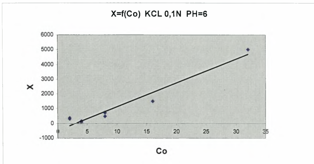
Διάγραμμα 3.1-3: Η προσρόφηση του καδμίου X (μg Cd/g γκαϊτίτη) σε συνάρτηση με την αρχική συγκέντρωση του καδμίου Co (μg Cd/ml διαλύματος) σε pH=6 και ηλεκτρολύτη KCl 0,1N.
