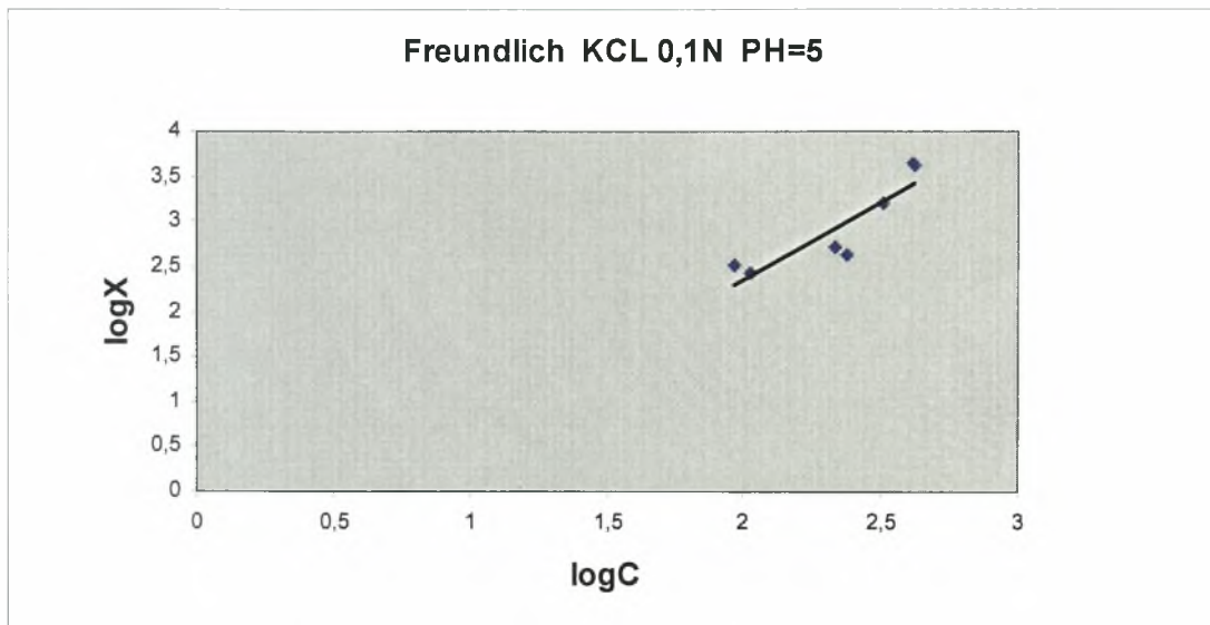
Διάγραμμα 3.3-2: Ο λογάριθμος του ποσού που προσροφάται σε συνάρτηση με τον λογάριθμο της συγκέντρωσης ισορροπίας σε pH=5 και παρουσία ηλεκτρολύτη KCl=0,1N.
