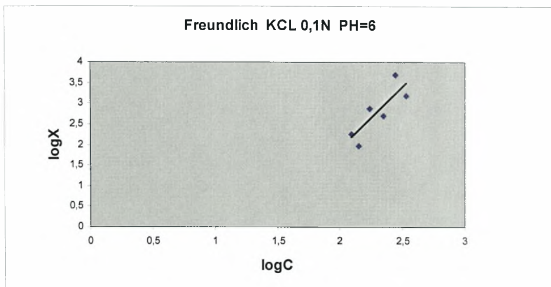
Διάγραμμα 3.3-3: Ο λογάριθμος του ποσού που προσροφάται σε συνάρτηση με τον λογάριθμο της συγκέντρωσης ισορροπίας σε pH=6 και παρουσία ηλεκτρολύτη KCl=0,1N.
