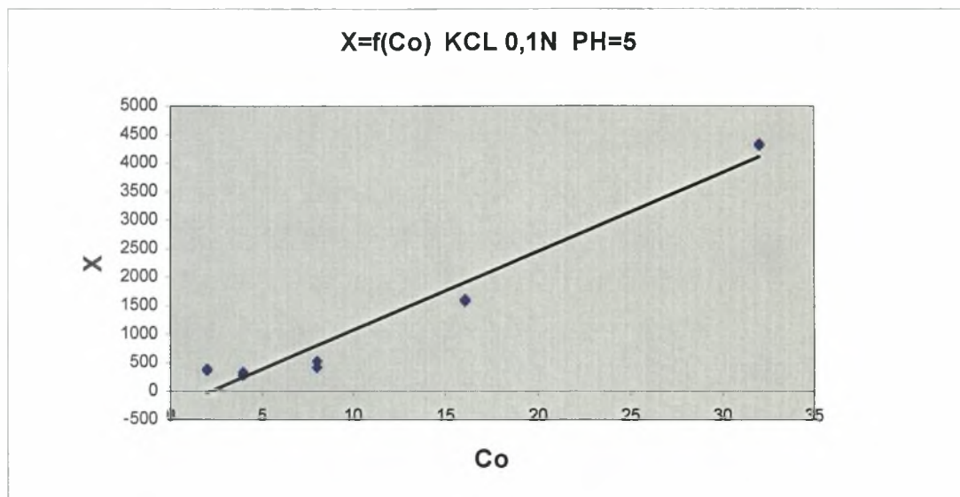
Διάγραμμα 3.1-2: Η προσρόφηση του καδμίου X (μg Cd/g γκαϊτίτη) σε συνάρτηση με την αρχική συγκέντρωση του καδμίου Co (μg Cd/ml διαλύματος) σε pH=5 και ηλεκτρολύτη KCl 0,1N.
