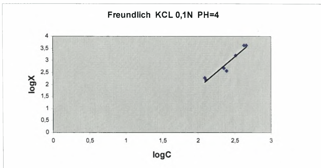
Διάγραμμα 3.3-1: Ο λογάριθμος του ποσού που προσροφάται σε συνάρτηση με τον λογάριθμο της συγκέντρωσης ισορροπίας σε pH=4 και παρουσία ηλεκτρολύτη KCl=0,1N.
