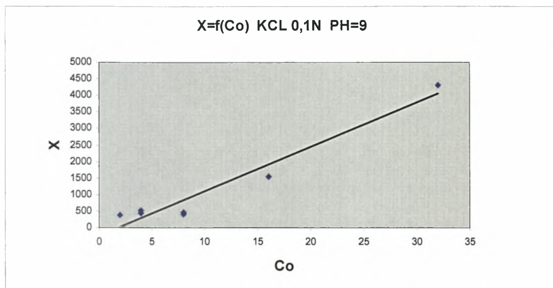
Διάγραμμα 3.1-6: προσρόφηση του καδμίου X (μg Cd/g γκαιτίτη) σε συνάρτηση με την αρχική συγκέντρωση του καδμίου Co (μg Cd/ml διαλύματος) σε pH=9 και ηλεκτρολύτη KCl 0,1N.
