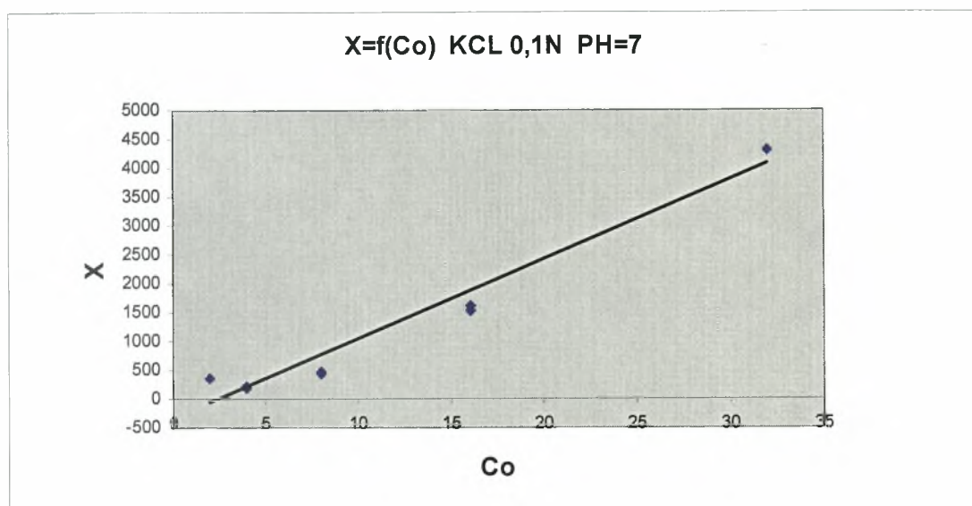
Διάγραμμα 3.1-4: Η προσρόφηση του καδμίου X ( \mu\text{g Cd/g} γκαϊτίτη) σε συνάρτηση με την αρχική συγκέντρωση του καδμίου Co ( \mu\text{g Cd/ml} διαλύματος) σε \text{pH}=7 και ηλεκτρολύτη \text{KCl } 0,1\text{N} .
