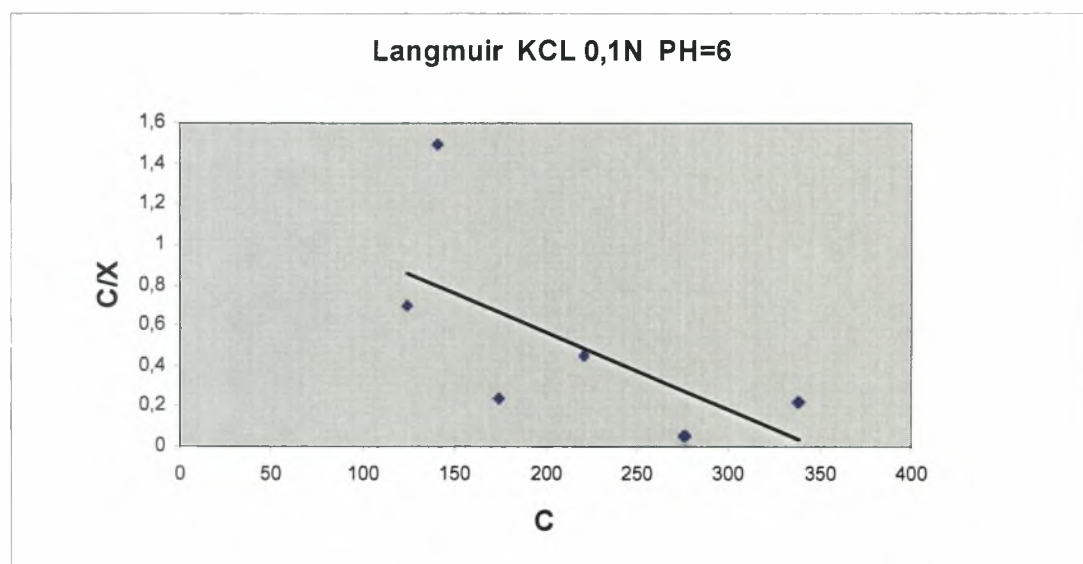
Διάγραμμα 3.2-3: Ο λόγος της συγκέντρωσης ισορροπίας (C mg/40ml) προς το ποσό της ουσίας που προσροφάται (X mg/g) σε συνάρτηση με τη συγκέντρωση ισορροπίας σε pH=6 και παρουσία ηλεκτρολύτη KCl=0,1N.
