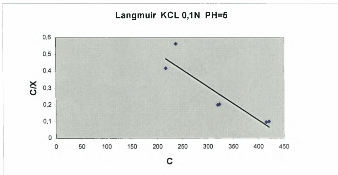
Διάγραμμα 3.2-2: Ο λόγος της συγκέντρωσης ισορροπίας ( C mg/40ml) προς το ποσό της ουσίας που προσροφάται ( X mg/g) σε συνάρτηση με τη συγκέντρωση ισορροπίας σε pH=5 και παρουσία ηλεκτρολύτη KCl=0,1N.
