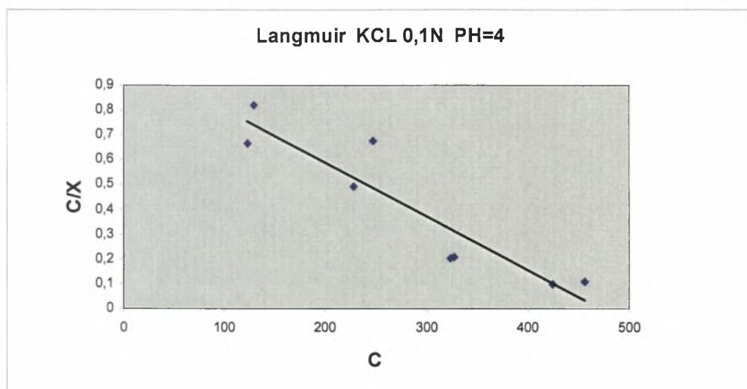
Διάγραμμα 3.2-1: Ο λόγος της συγκέντρωσης ισορροπίας ( C mg/40ml) προς το ποσό της ουσίας που προσροφάται ( X mg/g) σε συνάρτηση με τη συγκέντρωση ισορροπίας σε pH=4 και παρουσία ηλεκτρολύτη KCl=0,1N .
