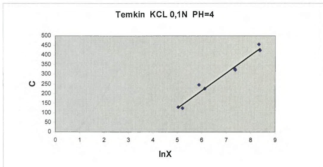
Διάγραμμα 3.4-1: Η συγκέντρωση ισορροπίας C (µg Cd/40ml) σε συνάρτηση με την ln του ποσού που προσροφάται σε pH=4 και παρουσία ηλεκτρολύτη KCl=0,1N.
