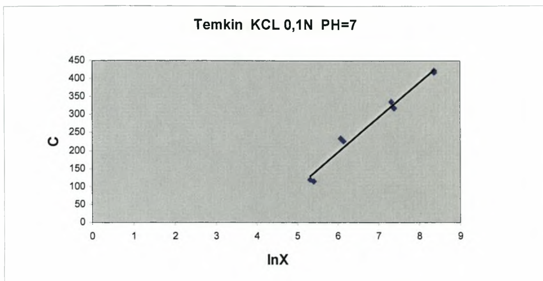
Διάγραμμα 3.4-4: Η συγκέντρωση ισορροπίας C (μg Cd/40ml) σε συνάρτηση με την ln του ποσού που προσροφάται σε pH=7 και παρουσία ηλεκτρολύτη KCl=0,1N.
