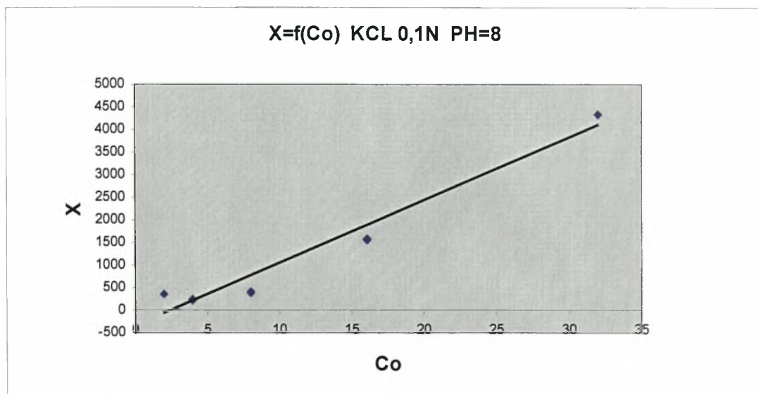
Διάγραμμα 3.1-5: Η προσρόφηση του καδμίου X ( \mu\text{g Cd/g} γκαϊτίτη) σε συνάρτηση με την αρχική συγκέντρωση του καδμίου Co ( \mu\text{g Cd/ml} διαλύματος) σε pH=8 και ηλεκτρολύτη KCl 0,1N.
