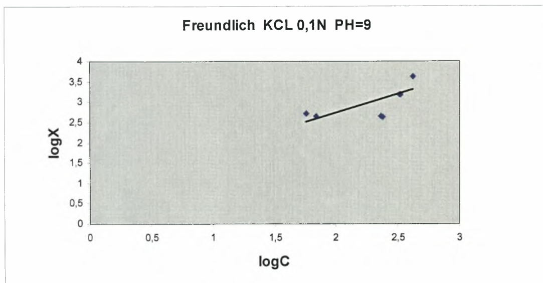
Διάγραμμα 3.3-6: Ο λογάριθμος του ποσού που προσροφάται σε συνάρτηση με τον λογάριθμο της συγκέντρωσης ισορροπίας σε pH=9 και παρουσία ηλεκτρολύτη KCl=0,1N.
