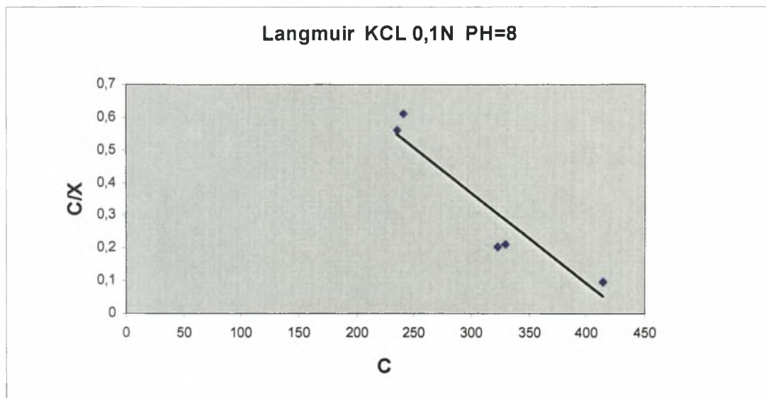
Διάγραμμα 3.2-5: Ο λόγος της συγκέντρωσης ισορροπίας ( C mg/40ml) προς το ποσό της ουσίας που προσροφάται ( X mg/g) σε συνάρτηση με τη συγκέντρωση ισορροπίας σε pH=8 και παρουσία ηλεκτρολύτη KCl=0,1N .
