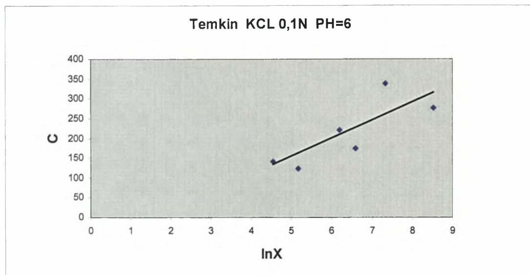
Διάγραμμα 3.4-3: Η συγκέντρωση ισορροπίας C (μg Cd/40ml) σε συνάρτηση με την ln του ποσού που προσροφάται σε pH=6 και παρουσία ηλεκτρολύτη KCl=0,1N.
