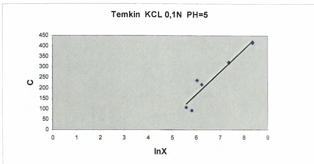
Διάγραμμα 3.4-2: Η συγκέντρωση ισορροπίας C (μg Cd/40ml) σε συνάρτηση με την ln του ποσού που προσροφάται σε pH=5 και παρουσία ηλεκτρολύτη KCl=0,1N.
