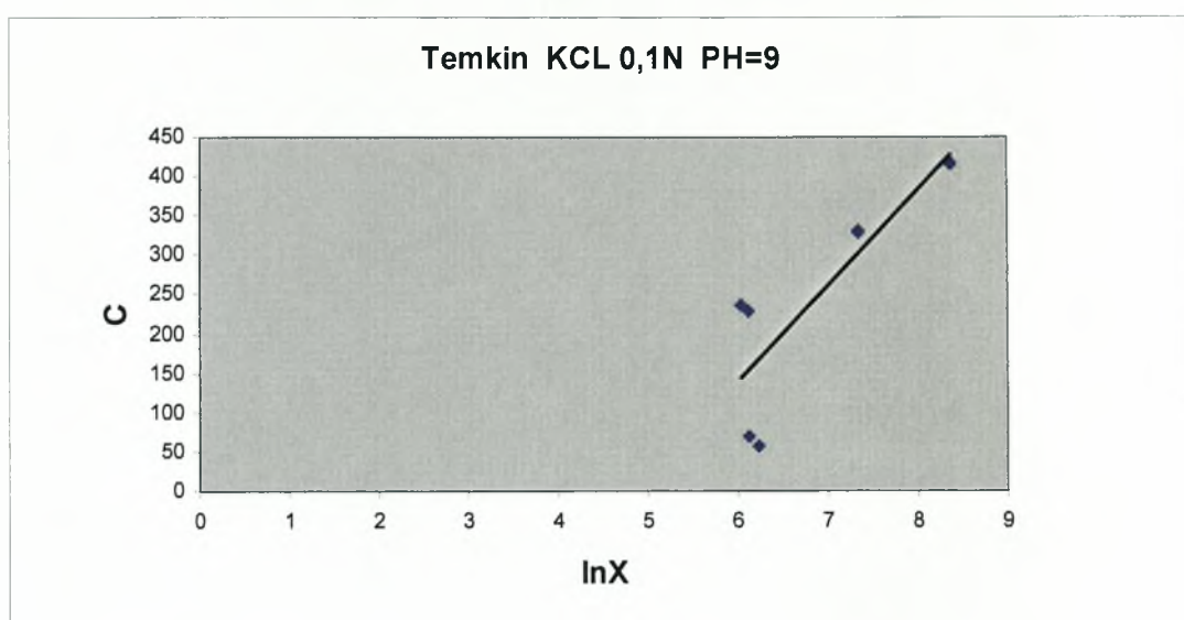
Διάγραμμα 3.4-6: Η συγκέντρωση ισορροπίας C (μg Cd/40ml) σε συνάρτηση με την ln του ποσού που προσροφάται σε pH=9 και παρουσία ηλεκτρολύτη KCl=0,1N.
