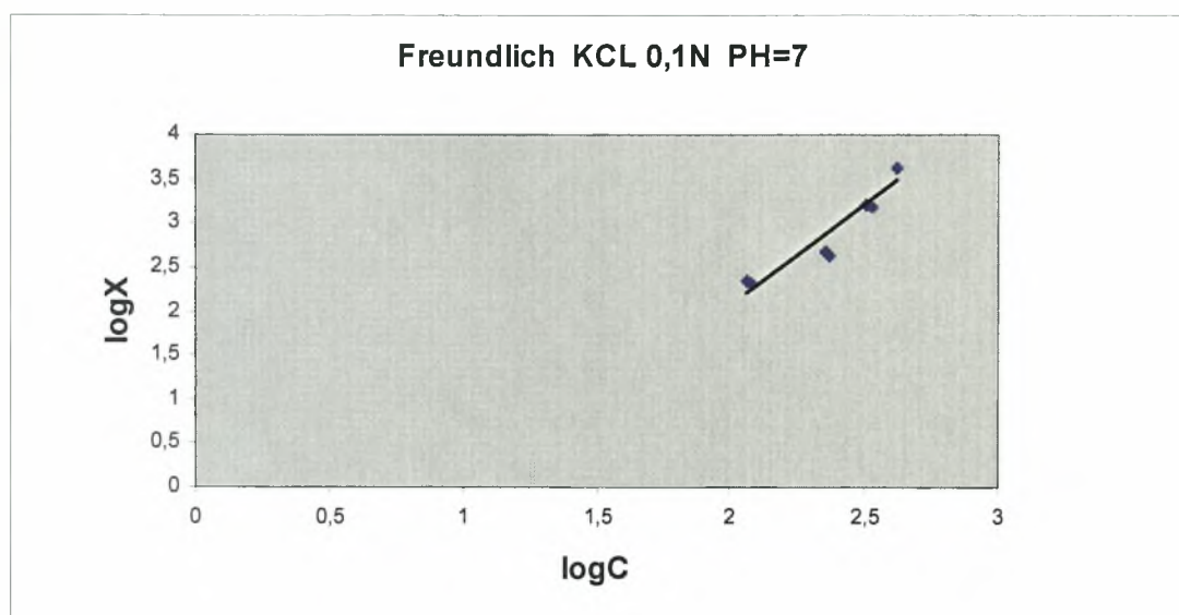
Διάγραμμα 3.3-4: Ο λογάριθμος του ποσού που προσροφάται σε συνάρτηση με τον λογάριθμο της συγκέντρωσης ισορροπίας σε pH=7 και παρουσία ηλεκτρολύτη KCl=0,1N.
