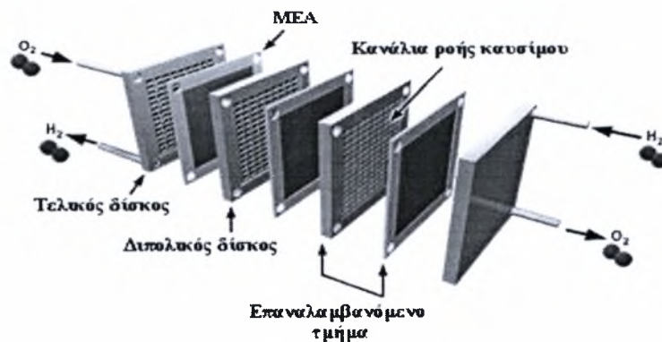
Σχήμα 3.6.1 Τυπική ηλεκτροχημική συστοιχία [14].
