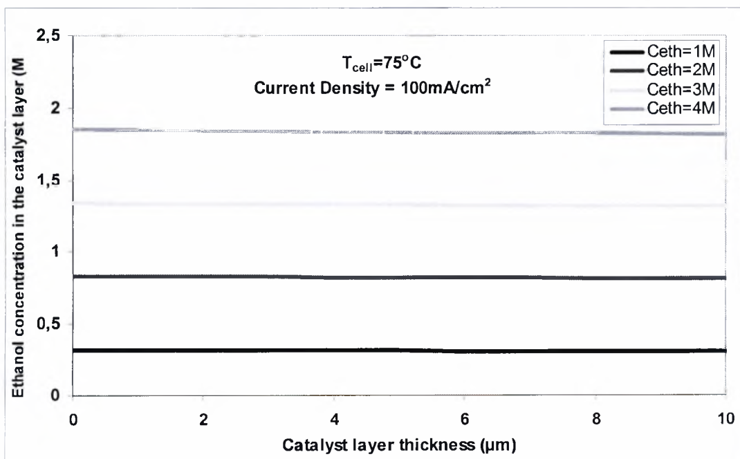
Σχήμα 5.2.11: Προβλεπόμενη συγκέντρωση αιθανόλης μέσα στον καταλύτη για διάφορες συγκεντρώσεις τροφοδοσίας και Current Density = 100 \text{ mA/cm}^2 .
