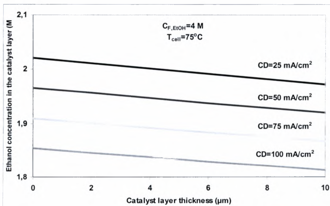
Σχήμα 5.2.9: Προβλεπόμενη συγκέντρωση αιθανόλης μέσα στον καταλύτη για διάφορες πυκνότητες ρεύματος C_{F,EtOH} = 4 \text{ M} .
