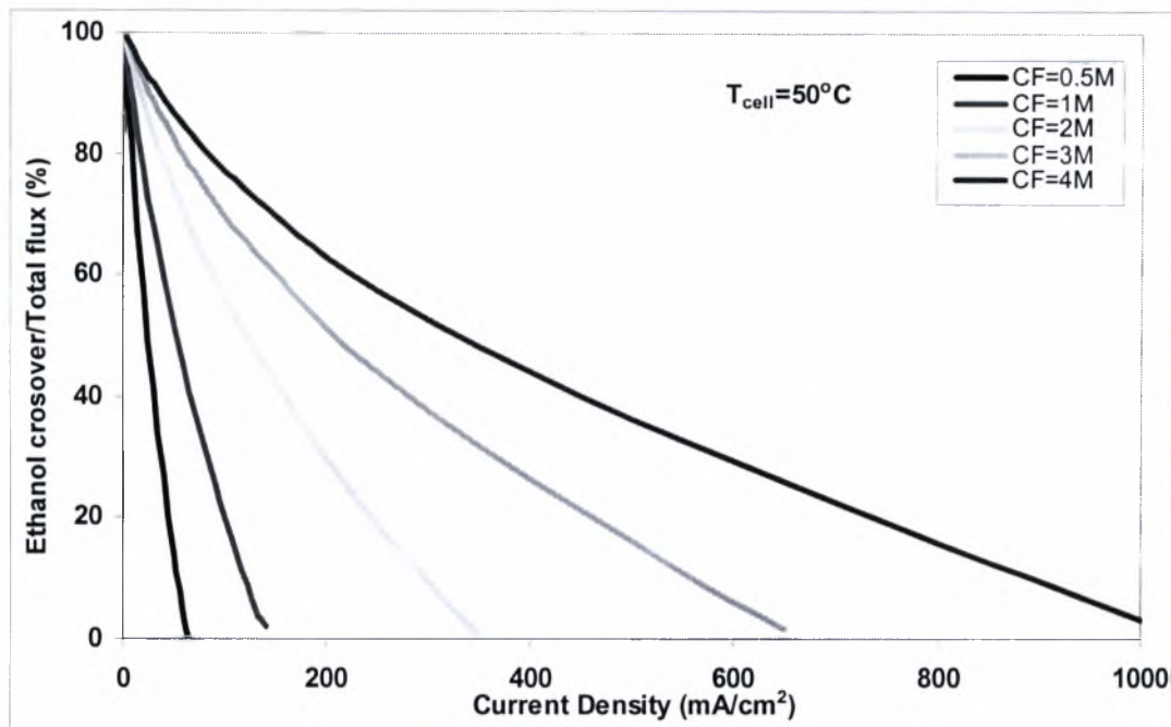
Σχήμα 5.2.35: Διαπερατότητα αιθανόλης ως ποσοστό του συνολικού ρυθμού της στο επίπεδο του καταλύτη για διάφορες πυκνότητες ρεύματος και διάφορες συγκεντρώσεις τροφοδοσίας, T cell =50°C.
