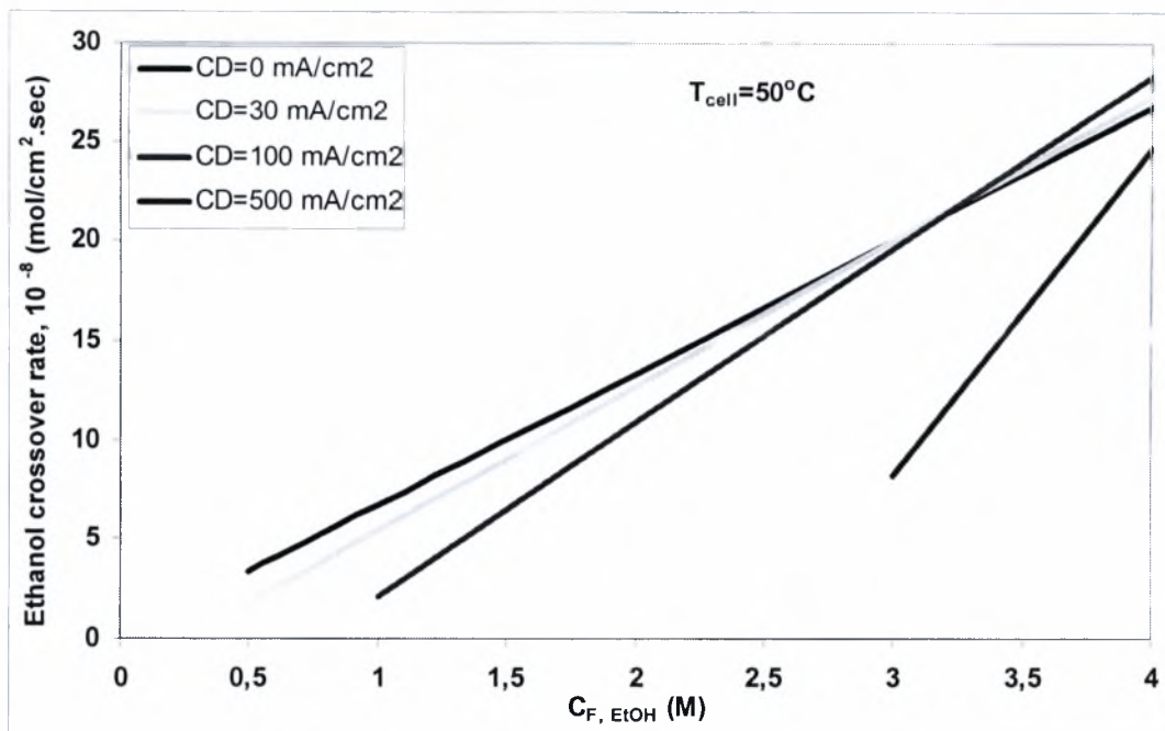
Σχήμα 5.2.41: Ρυθμός διαπερατότητας αιθανόλης συναρτήσει της τροφοδοτούμενη αιθανόλης για διάφορες πυκνότητες ρεύματος, T_{\text{cell}} = 50^\circ\text{C} .
