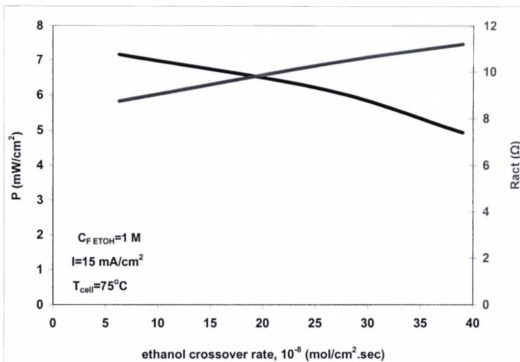
Σχήμα 5.2.50 : Μεταβολή της ισχύς και της αντίστασης του κελιού σε συνάρτηση με το ρυθμό της διαπερατότητας της αιθανόλης, I = 15 \text{ mA}/\text{cm}^2 .
