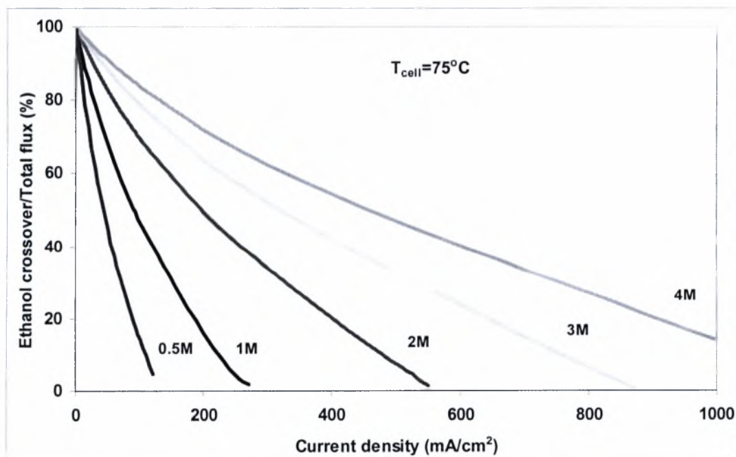
Σχήμα 5.2.34: Διαπερατότητα αιθανόλης ως ποσοστό του συνολικού ρυθμού της στο επίπεδο του καταλύτη για διάφορες πυκνότητες ρεύματος και διάφορες συγκεντρώσεις τροφοδοσίας, T_{cell}=75^{\circ}C .
