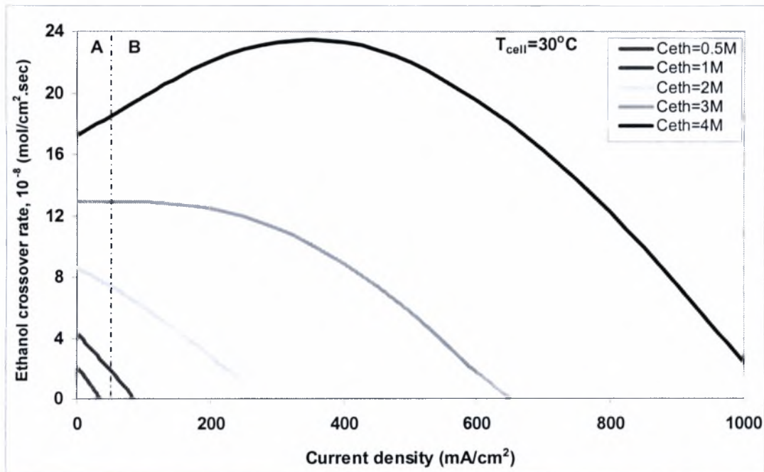
Σχήμα 5.2.32: Επίδραση της πυκνότητας ρεύματος στη διαπερατότητα της αιθανόλης για διάφορες συγκεντρώσεις τροφοδοσίας, T_{cell}=30^{\circ}C .
