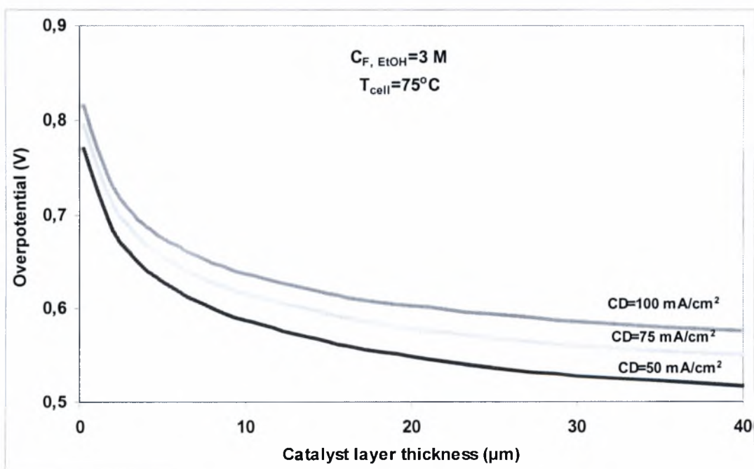
Σχήμα 5.2.15: Επίδραση του πάχους του καταλύτη στην υπέρταση ανόδου, C_{F, \text{EtOH}} = 3 \text{ M} , T_{\text{cell}} = 75^\circ\text{C} .
