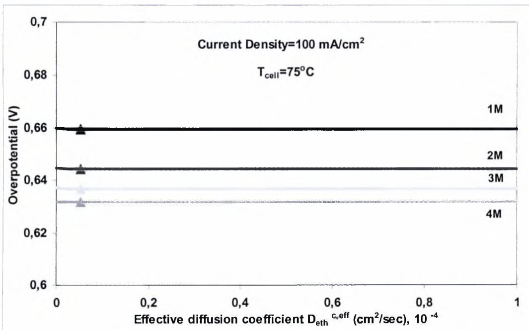
Σχήμα 5.2.22: Μεταβολή της υπέρτασης στην άνοδο συναρτήσει του αποδοτικού συντελεστή διάχυσης, D_{\text{ethyl}}^{c,\text{eff}} , \text{CD} = 100 \text{ mA}/\text{cm}^2 , T_{\text{cell}} = 75^\circ\text{C} .
