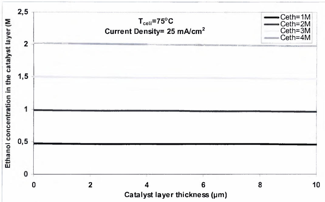
Σχήμα 5.2.10: Προβλεπόμενη συγκέντρωση αιθανόλης μέσα στον καταλύτη για διάφορες συγκεντρώσεις τροφοδοσίας, Current Density = 25 \text{ mA/cm}^2 .
