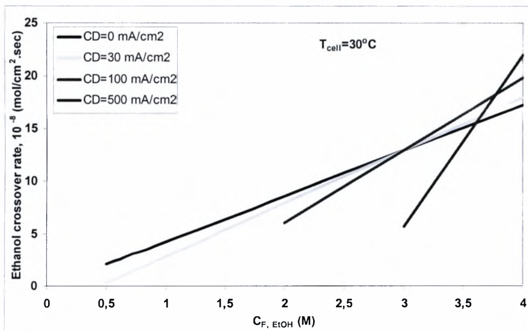
Σχήμα 5.2.42: Ρυθμός διαπερατότητας της αιθανόλης συναρτήσει της τροφοδοτούμενης αιθανόλης για διάφορες πυκνότητες ρεύματος, T_{\text{cell}} = 30^\circ\text{C} .
