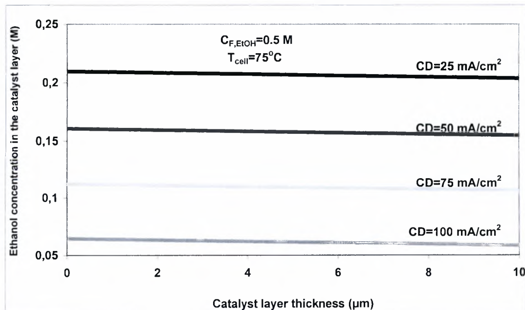
Σχήμα 5.2.5: Προβλεπόμενη συγκέντρωση αιθανόλης μέσα στον καταλύτη για διάφορες πυκνότητες ρεύματος, C_{F,EtOH} = 0.5 \text{ M} .
