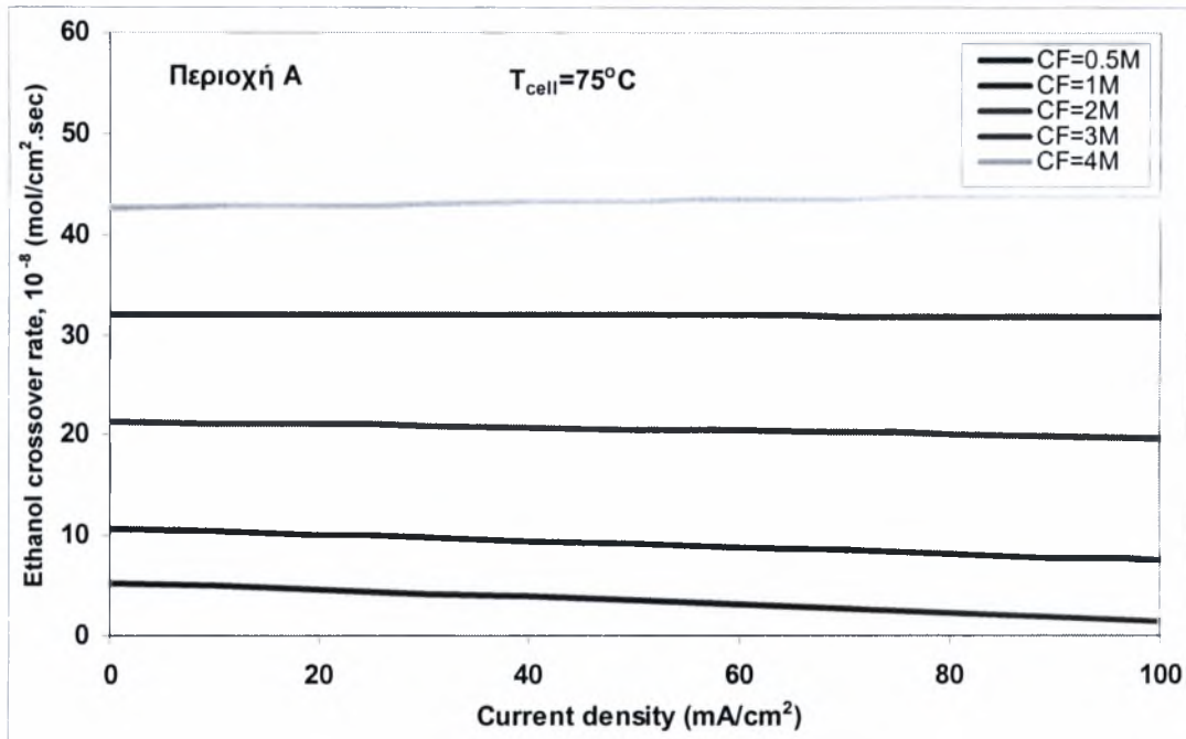
Σχήμα 5.2.29: Επίδραση της πυκνότητας ρεύματος (~ 100 mA/cm 2 ) στη διαπερατότητα της αιθανόλης για διάφορες συγκεντρώσεις τροφοδοσίας, T_{cell}=75 °C.
