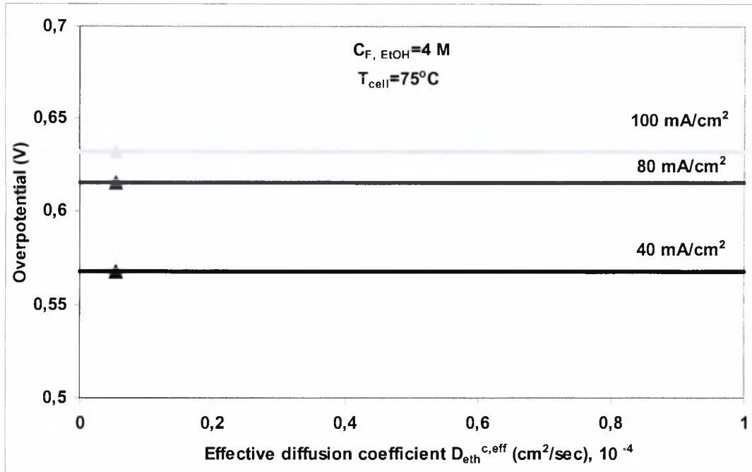
Σχήμα 5.2.21: Μεταβολή της υπέρτασης στην άνοδο συναρτήσει του αποδοτικού συντελεστή διάχυσης, D_{\text{ethyl}}^{c,\text{eff}} για διάφορες πυκνότητες ρεύματος. C_{F, \text{EtOH}} = 4 \text{ M} , T_{\text{cell}} = 75^\circ\text{C} .
