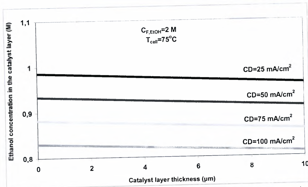
Σχήμα 5.2.7: Προβλεπόμενη συγκέντρωση αιθανόλης μέσα στον καταλύτη για διάφορες πυκνότητες ρεύματος, C_{F,EtOH} = 2 \text{ M} .
