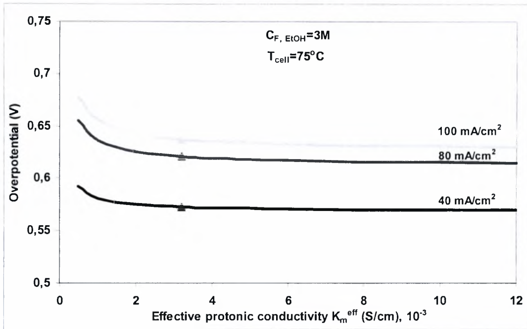
Σχήμα 5.2.25: μεταβολή της υπέρτασης ανόδου σε σχέση με τον αποδοτικό συντελεστή πρωτονιακής αγωγιμότητας, K_m^{eff} για διάφορες πυκνότητες ρεύματος. C_{F, EtOH} = 3 M , T_{cell} = 75^\circ C .
