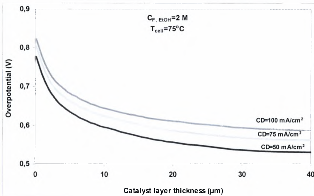
Σχήμα 5.2.14: Επίδραση του πάχους του καταλύτη στην υπέρταση ανόδου, C_{F, \text{EtOH}} = 2 \text{ M} , T_{\text{cell}} = 75^\circ\text{C} .
