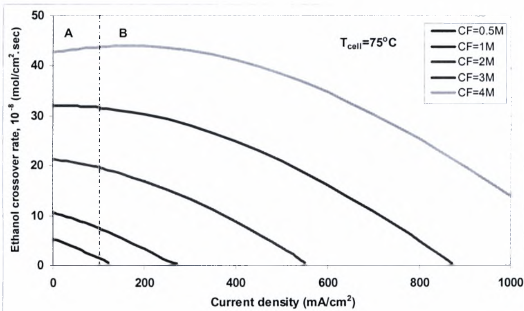
Σχήμα 5.2.28: Επίδραση της πυκνότητας ρεύματος στη διαπερατότητα της αιθανόλης για διάφορες συγκεντρώσεις τροφοδοσίας, T_{cell}=75\text{ }^{\circ}\text{C} .
