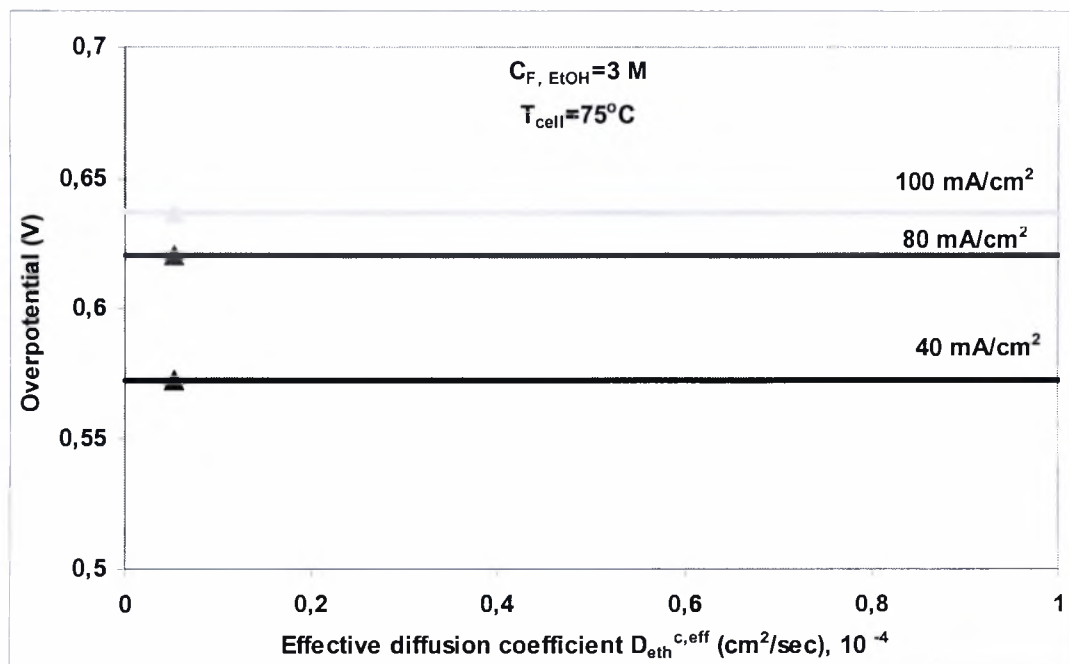
Σχήμα 5.2.20: Μεταβολή της υπέρτασης στην άνοδο συναρτήσει του αποδοτικού συντελεστή διάχυσης, D_{\text{ethyl}}^{c,\text{eff}} για διάφορες πυκνότητες ρεύματος. C_{\text{F, EtOH}} = 3 \text{ M} , T_{\text{cell}} = 75^\circ\text{C} .
