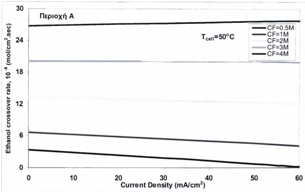
Σχήμα 5.2.31: Επίδραση της πυκνότητας ρεύματος ( \sim 60 mA/cm 2 ) στη διαπερατότητα της αιθανόλης για διάφορες συγκεντρώσεις τροφοδοσίας, T_{cell}=50^{\circ}C .
