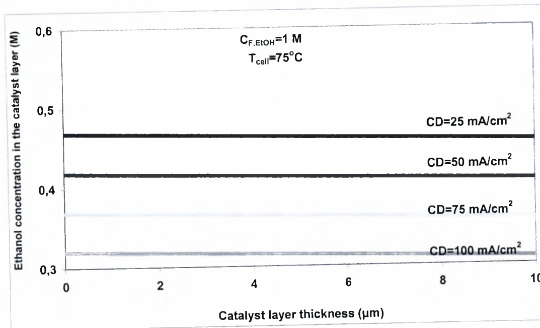
Σχήμα 5.2.6: Προβλεπόμενη συγκέντρωση αιθανόλης μέσα στον καταλύτη για διάφορες πυκνότητες ρεύματος, C_{F,EtOH} = 1 \text{ M} .
