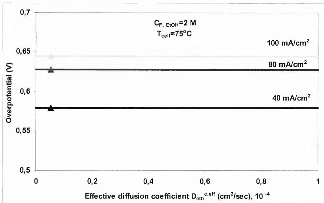
Σχήμα 5.2.19: Μεταβολή της υπέρτασης στην άνοδο συναρτήσει του αποδοτικού συντελεστή διάχυσης, D_{\text{ethyl}}^{c,\text{eff}} για διάφορες πυκνότητες ρεύματος. C_{\text{F, EtOH}} = 2 \text{ M} , T_{\text{cell}} = 75^\circ\text{C} .
