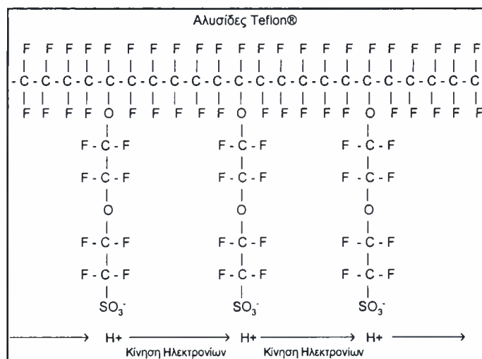
Σχήμα 3.2.1.1: Αλυσίδες Nafion [7].
