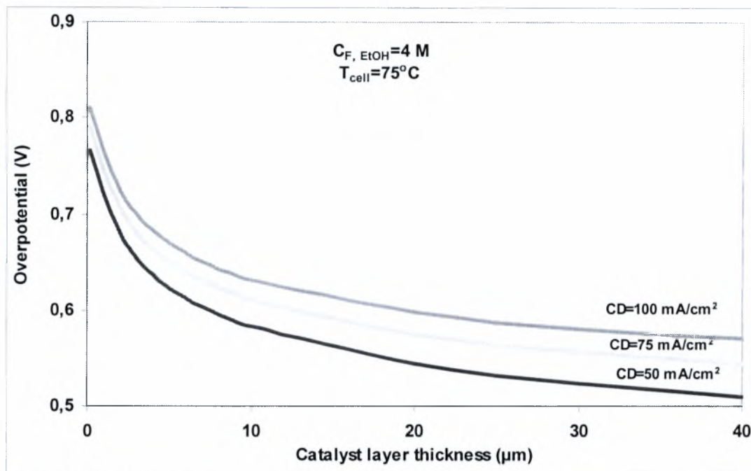
Σχήμα 5.2.16: Επίδραση του πάχους του καταλύτη στην υπέρταση ανόδου, C_{F, EtOH} = 4 M , T_{cell} = 75^{\circ}C .
