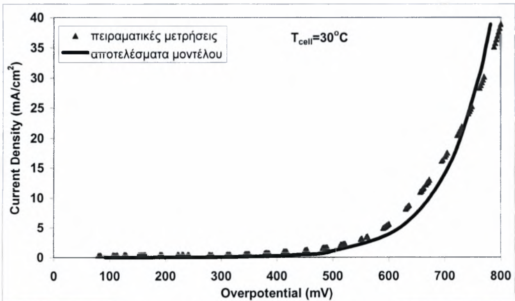
Σχήμα 5.2.3: Ανοδική υπέρταση DEFC. Πειραματικές συνθήκες: T cell = 30°C, C F , C F, EtOH = 1M [57].
