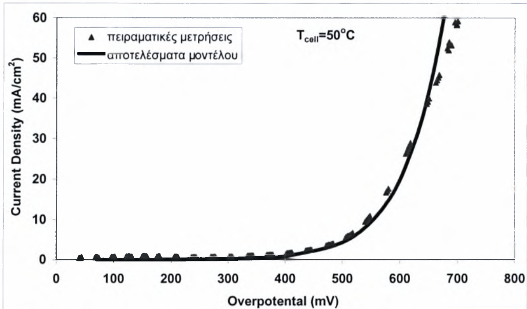
Σχήμα 5.2.2: Ανοδική υπέρταση DEFC. Πειραματικές συνθήκες: T cell = 50°C, C F , C F, EtOH = 1M [57].
