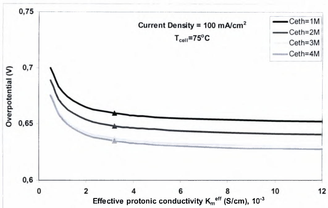
Σχήμα 5.2.27: μεταβολή της υπέρτασης ανόδου σε σχέση με τον αποδοτικό συντελεστή πρωτονιακής αγωγιμότητας, K_m^{eff} για πυκνότητα ρεύματος 100 mA/cm 2 και διάφορες συγκεντρώσεις τροφοδοσίας.
