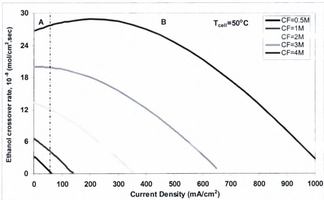
Σχήμα 5.2.30: Επίδραση της πυκνότητας ρεύματος στη διαπερατότητα της αιθανόλης για διάφορες συγκεντρώσεις τροφοδοσίας, T_{cell}=50 °C.
