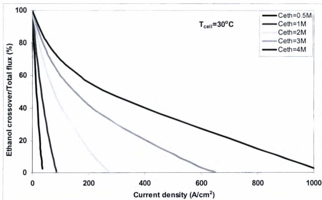
Σχήμα 5.2.36: Διαπερατότητα αιθανόλης ως ποσοστό του συνολικού ρυθμού της στο επίπεδο του καταλύτη για διάφορες πυκνότητες ρεύματος και διάφορες συγκεντρώσεις τροφοδοσίας, T cell =30°C.
