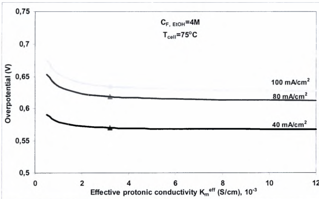
Σχήμα 5.2.26: μεταβολή της υπέρτασης ανόδου σε σχέση με τον αποδοτικό συντελεστή πρωτονιακής αγωγιμότητας, K_m^{eff} για διάφορες πυκνότητες ρεύματος. C_{F, EtOH} = 4 M , T_{cell} = 75^\circ C .
