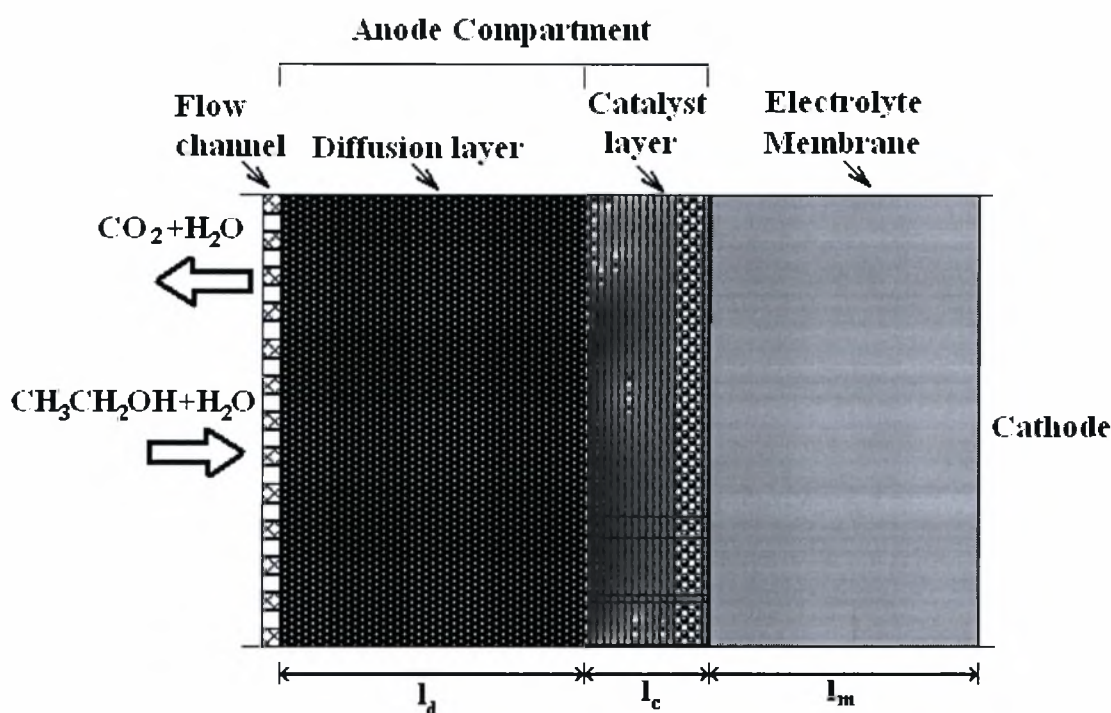
Σχήμα 4.1.1: Σχηματική απεικόνιση της άνοδου του DEFC που χρησιμοποιήθηκε στο μοντέλο.
