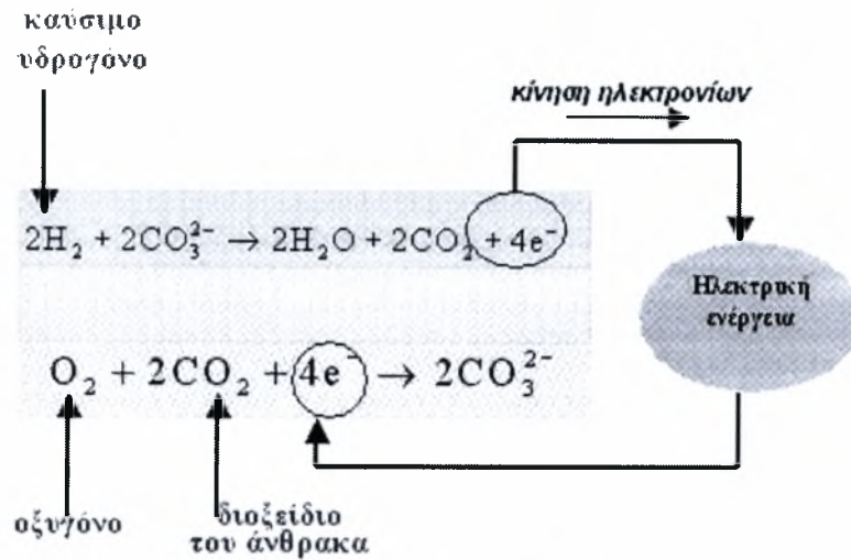
Σχήμα 2.6.4.1: Αρχή λειτουργίας ενός MCFC.
