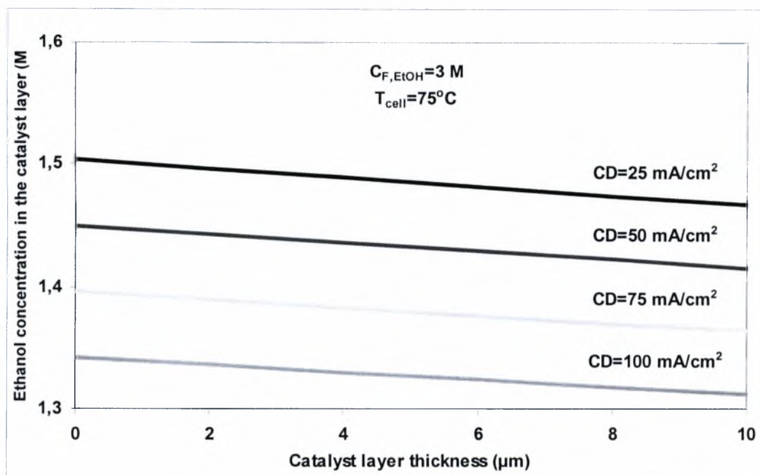
Σχήμα 5.2.8: Προβλεπόμενη συγκέντρωση αιθανόλης μέσα στον καταλύτη για διάφορες πυκνότητες ρεύματος, C_{F,EtOH} = 3 \text{ M} .
