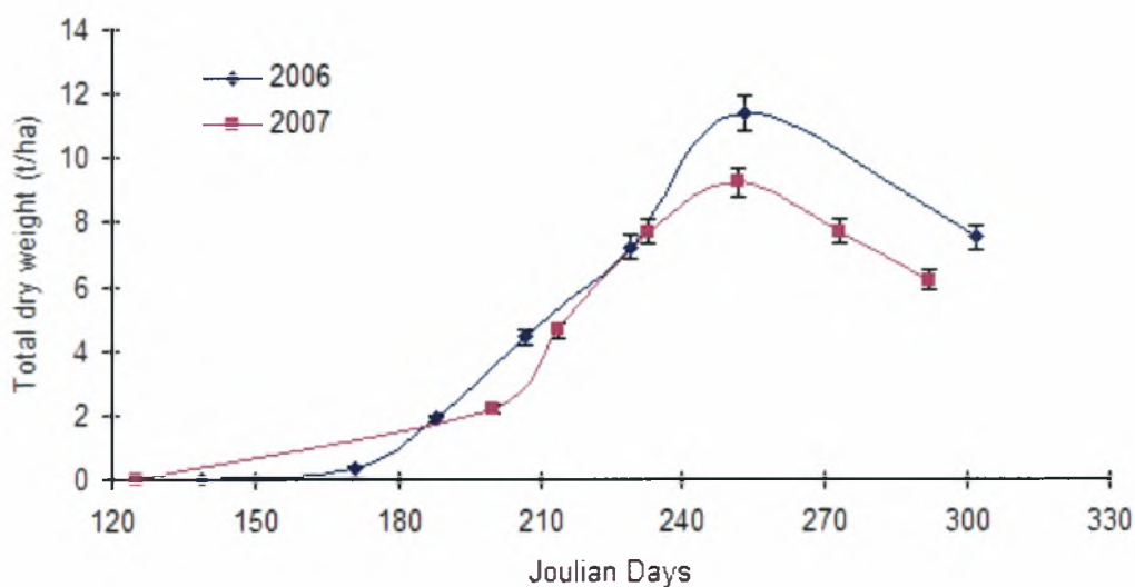
Σχήμα 3. Αύξηση σε ολική ξηρή βιομάζα (t/ha) της καλλιέργειας βαμβακιού στον Παλαμά – Καρδίτσας το 2006 και το 2007. Τα δεδομένα αποτελούν μέσους όρους όλων των πειραματικών τεμαχίων ( \pm απόκλιση μέσου όρου) για κάθε έτος.
