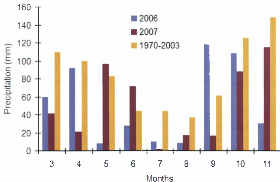
Σχήμα 2. Αθροιστική μηνιαία βροχόπτωση το 2006 και το 2007 σε σύγκριση με την μέση κλιματική τιμή των τελευταίων 30 ετών στην περιοχή του Παλαμά. Δεδομένα μέσης κλιματικής τιμής είναι ο μέσος όρος από Τρίκαλα και Λάρισα (πηγή: ΕΜΥ).
