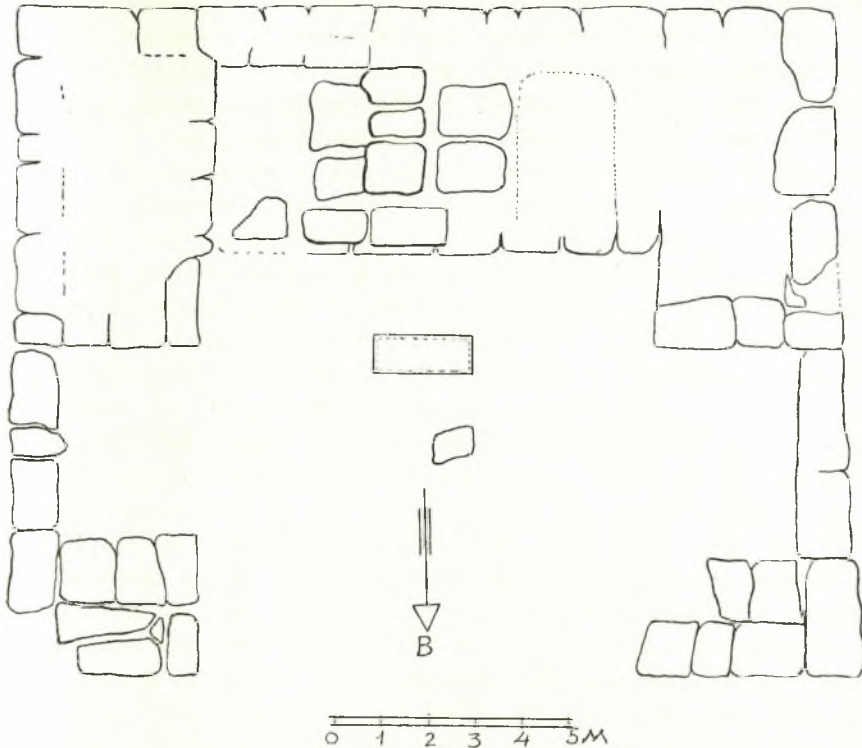
Εἰκ. 2. Ψυχικό. Τὸ σχέδιον τοῦ βομοειδοῦς οἰκοδομήματος.
