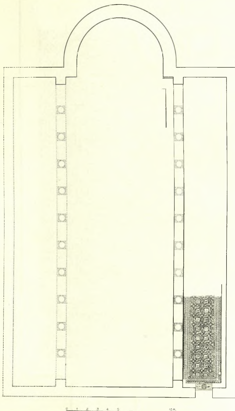
Εικ. 4. Κάτοπις τής βασιλικής Α τής Άμφιπόλεως.
