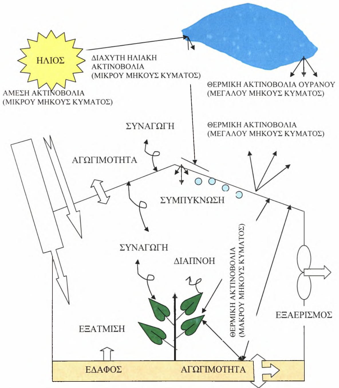
Εικόνα 2.1 Ανταλλαγές ενέργειας του θερμοκηπίου με το περιβάλλον
