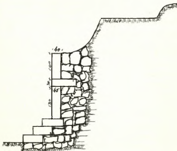
Τομή ζ - ζ.
