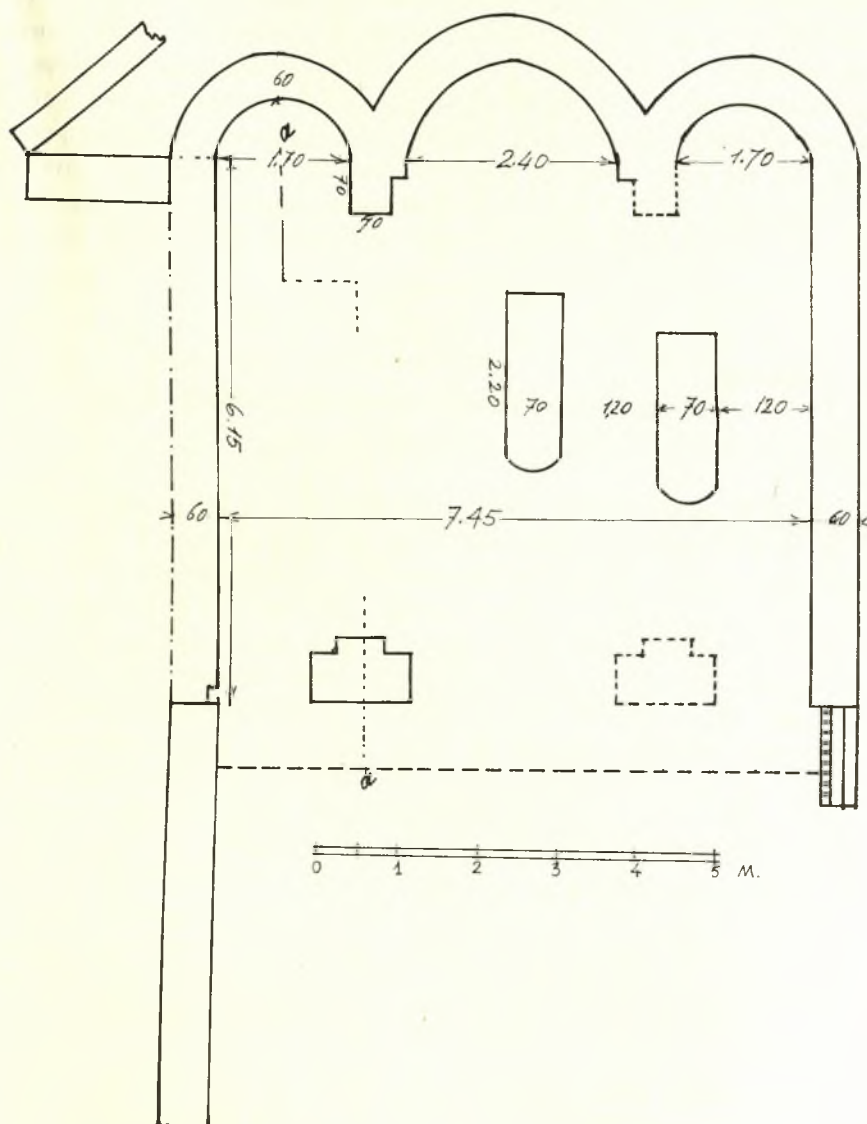
Είχ. 2. Κάτοπις τοῦ χριςτιανικοῦ ναοῦ.
