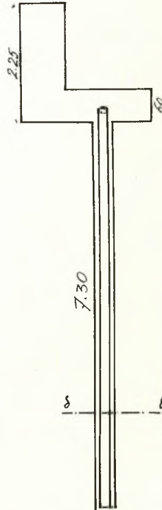
Κάτοπις θυσιαστηρίου.
