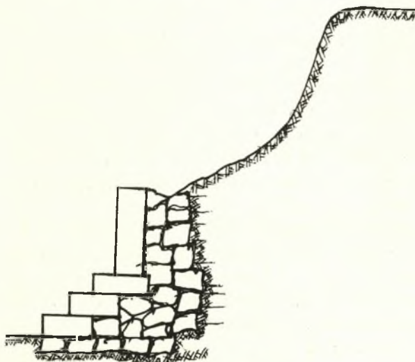
Τομή η - η.
