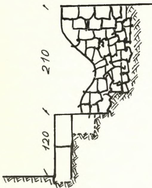
Τομή β - β.
