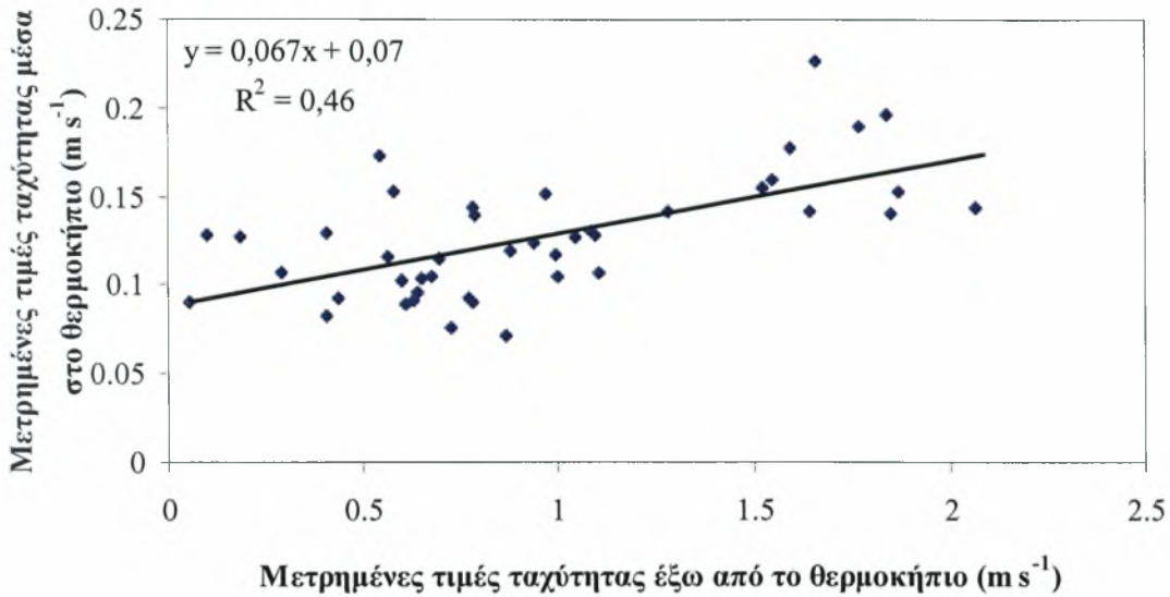
Σχήμα 4.1 Σχέση μεταξύ των μετρημένων τιμών της ταχύτητας του άνεμου μέσα ( u_i ) και έξω ( u_o ) από το θερμοκήπιο
