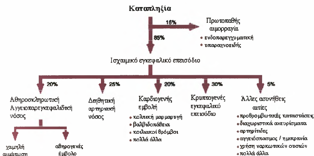
Σχήμα 11. Ταξινόμηση του εγκεφαλικού επεισοδίου 116 .
