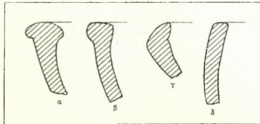
Εἰκ. 4. Χαρακτηριστικαὶ τομαὶ χειλέων πρωτοελλαδικῶν ἀγγείων (1:2).
