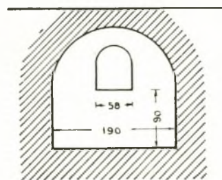
ΕΓΚΑΡΣΙΑ ΤΟΜΗ
