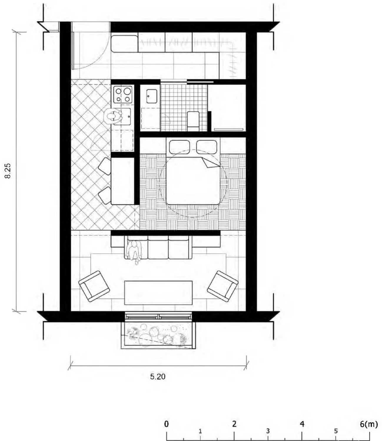
Κάτοψη τυπικού διαμερίσματος Β' ορόφου
