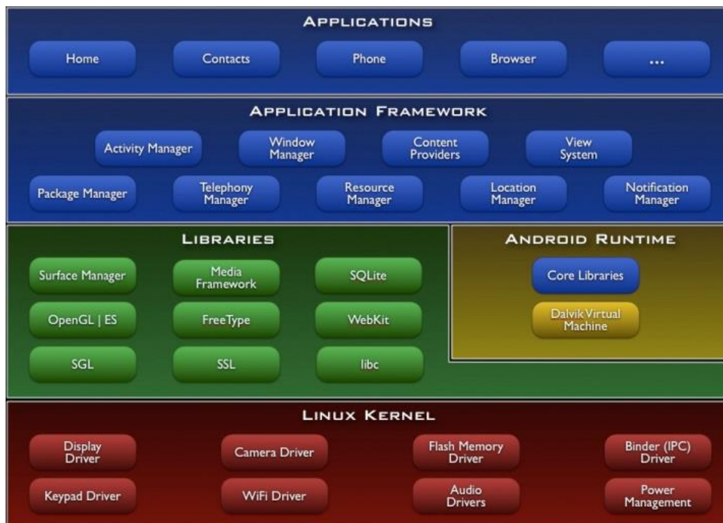
Εικόνα 1: Android layers
