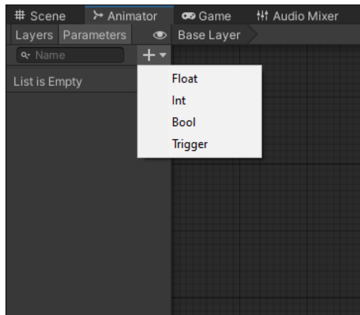
Parameter Types
