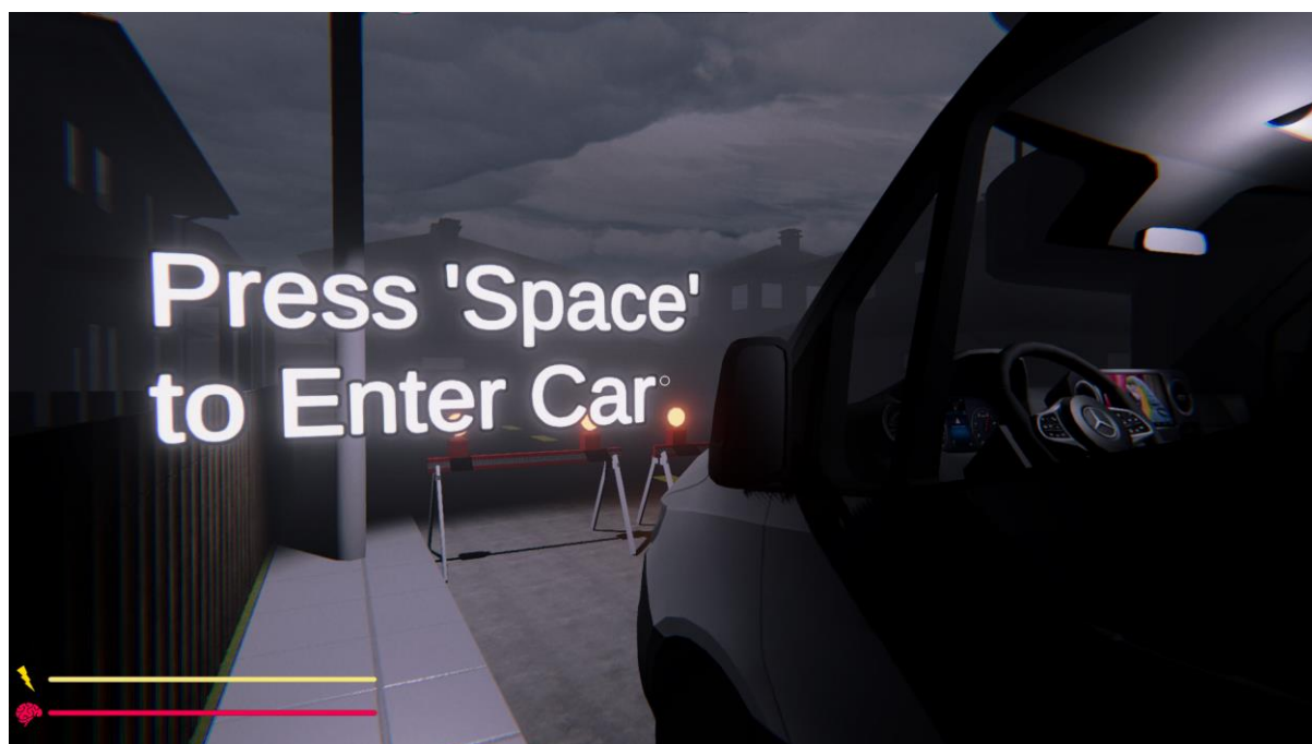
Van EndGame
