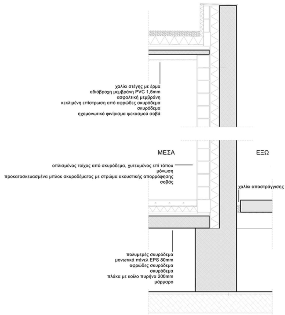
ΚΑΤΑΣΚΕΥΑΣΤΙΚΕΣ ΛΕΠΤΟΜΕΡΕΙΕΣ - ΑΙΘΟΥΣΑ ΤΕΛΕΤΩΝ
