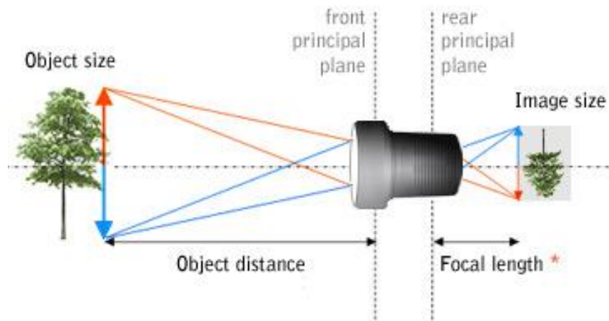
Εικόνα15. Distance Calculation from Camera.
