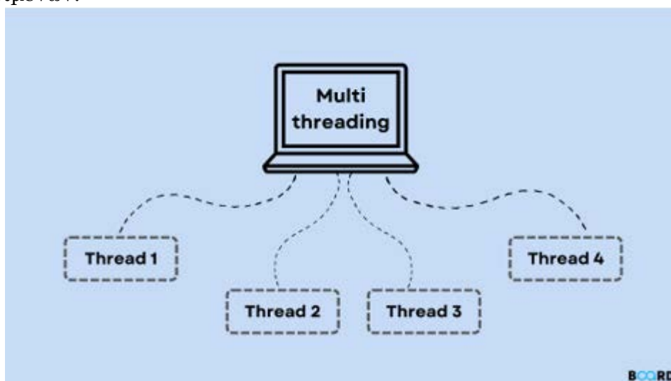
Εικόνα20. Multi-Threading Visualization.
