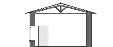
ΤΟΜΗ ΔΔ AM6239
